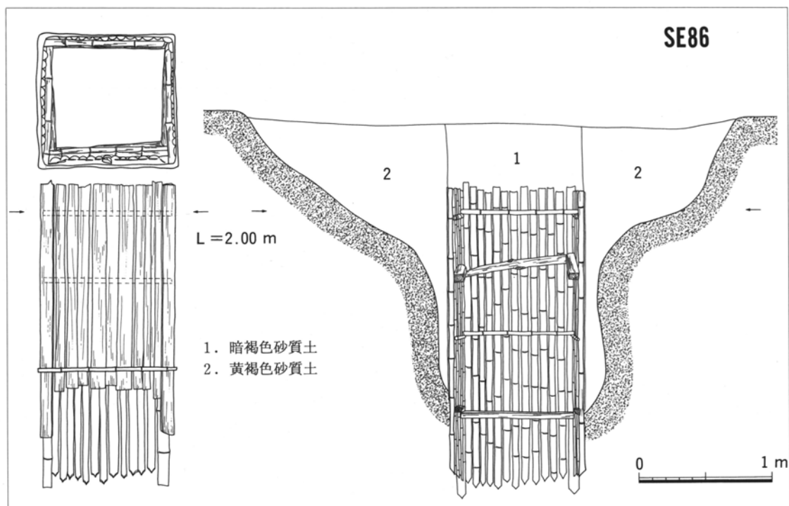
第15図 井戸実測図(6)
