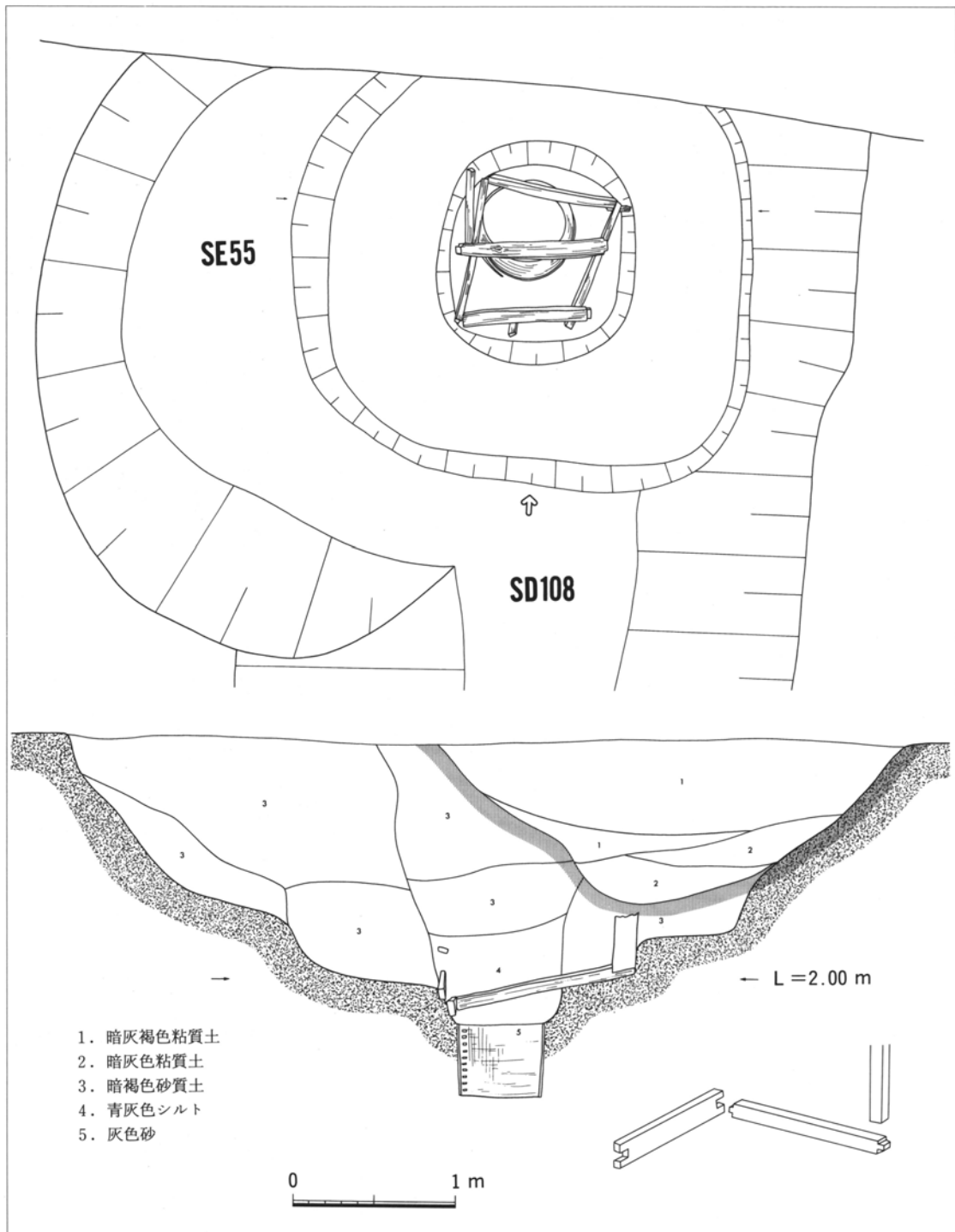
第11図 井戸実測図(2)
