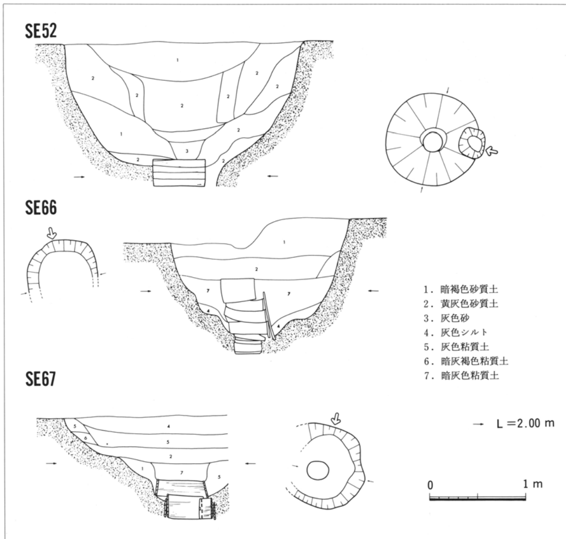
第10図 井戸実測図(1)
