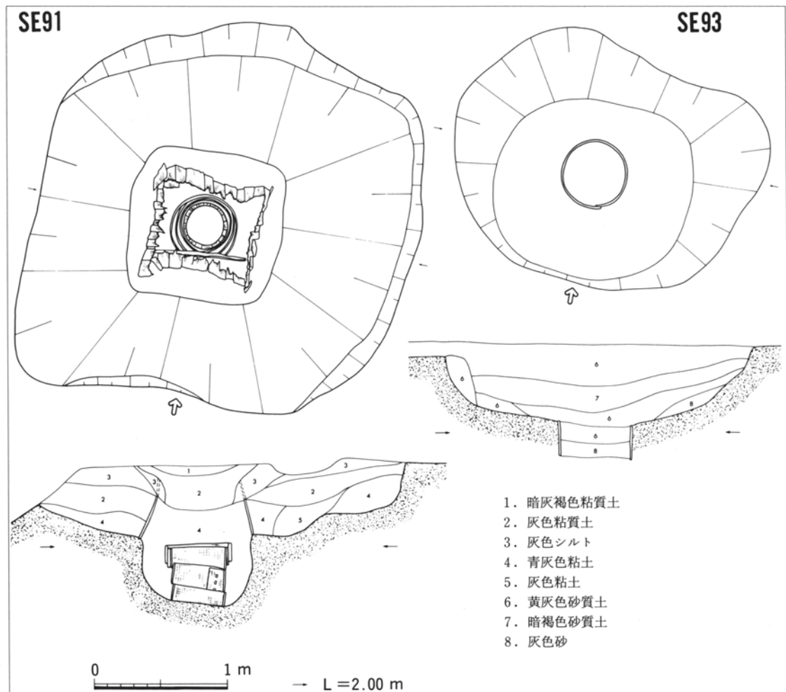
第13図 井戸実測図(4)
