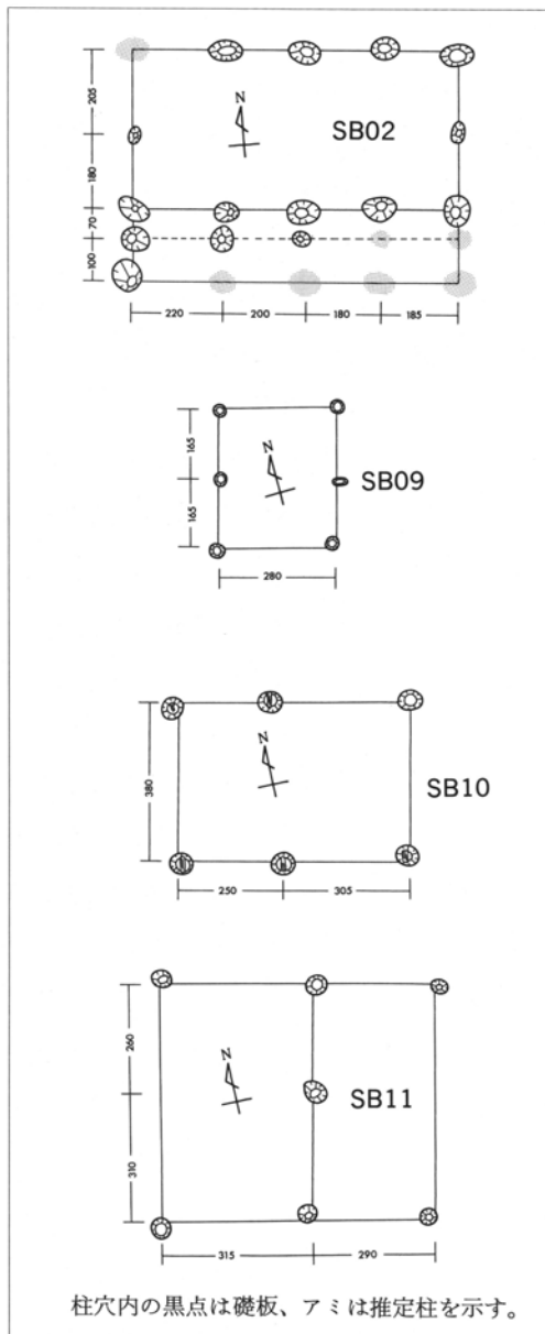
第6図 建物跡模式図(1) (単位は cm)
