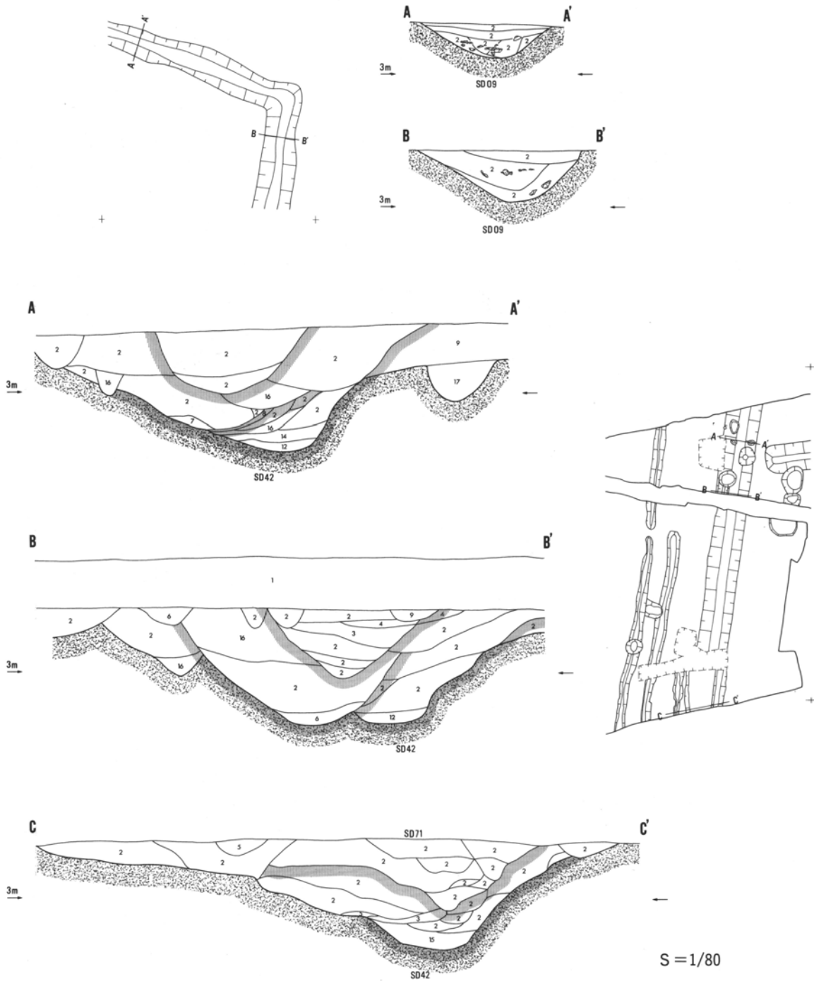
第7図 溝セクション図(1)
