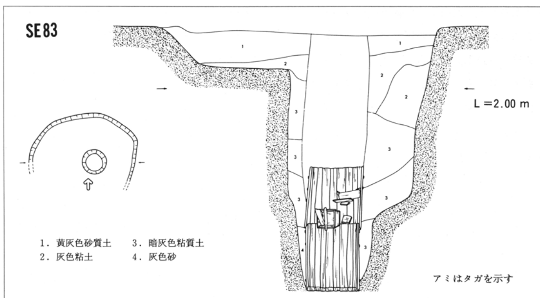
第28図 井戸実測図(13)
