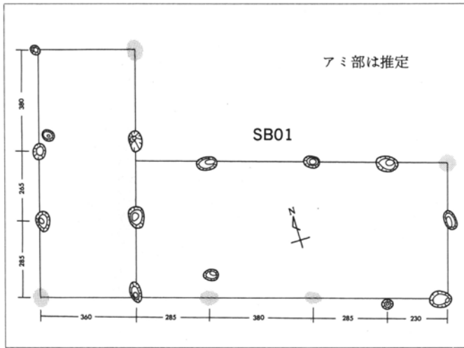
第19図 建物跡模式図(2) (単位は cm)
