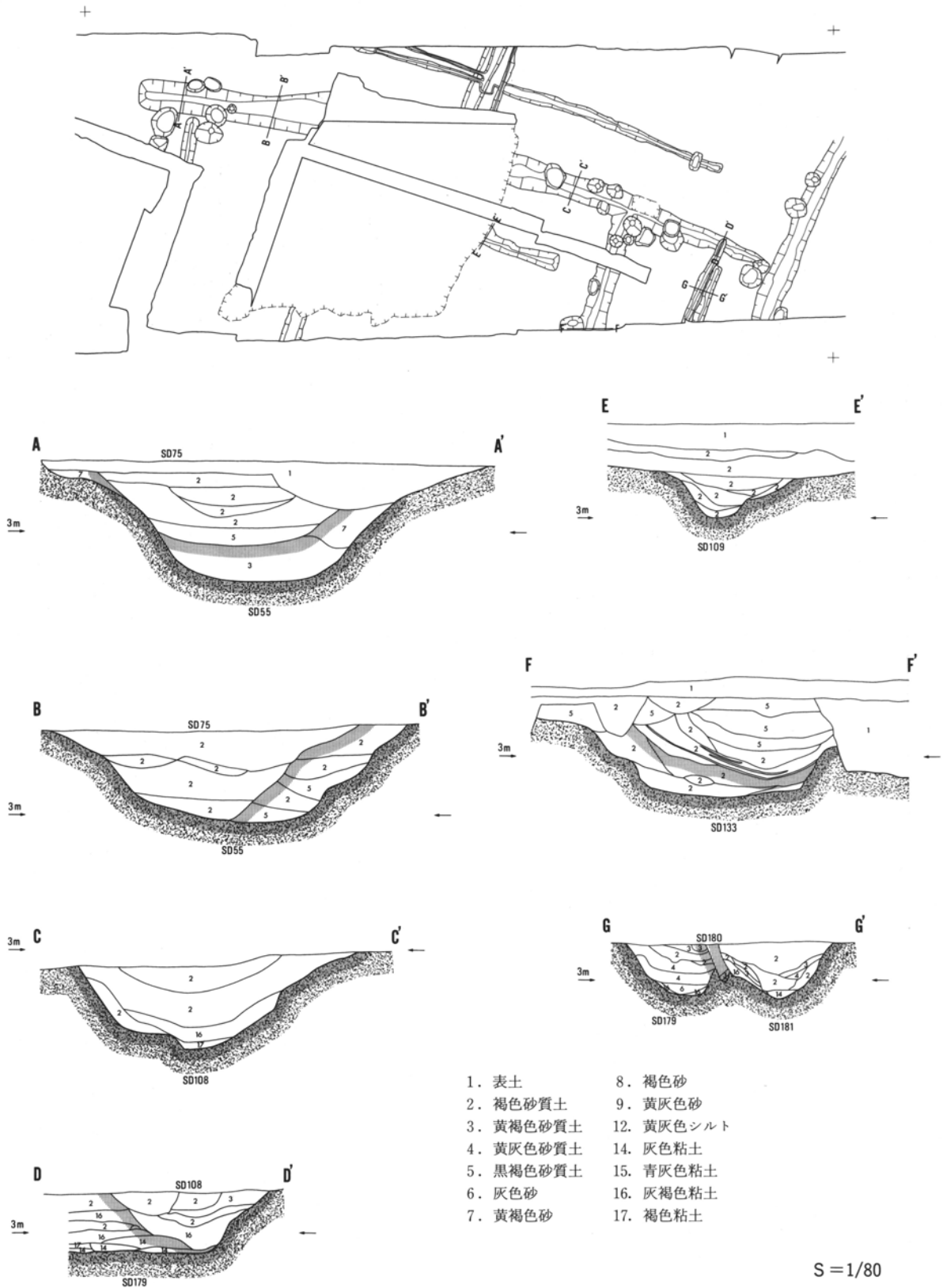
第8図 溝セクション図(2)
