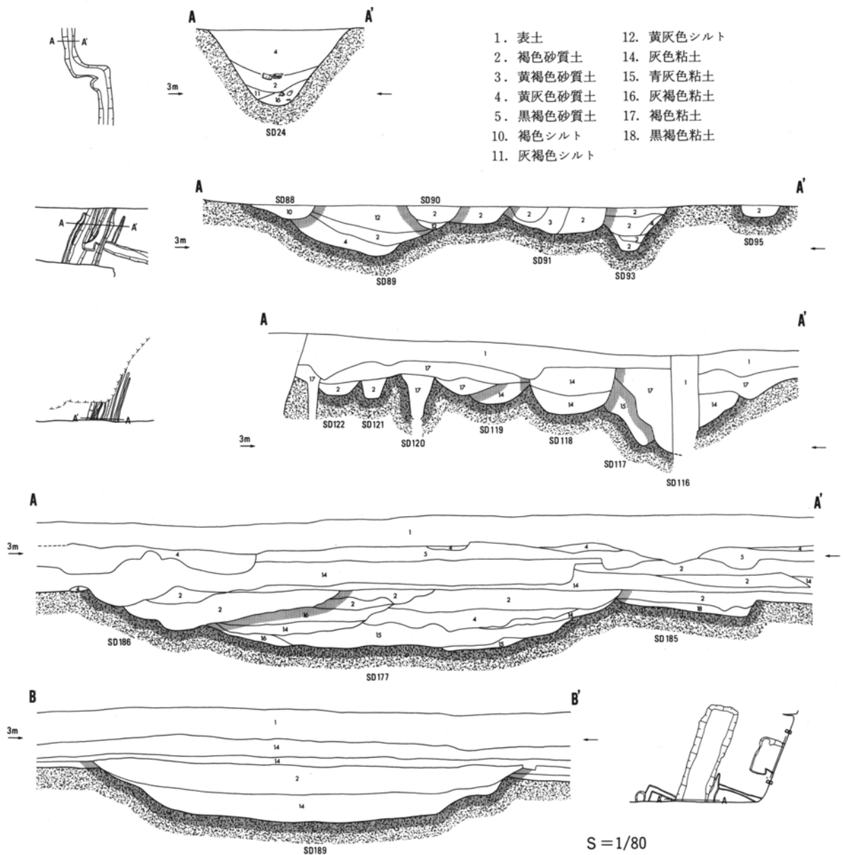
第21図 溝セクション図(4)
