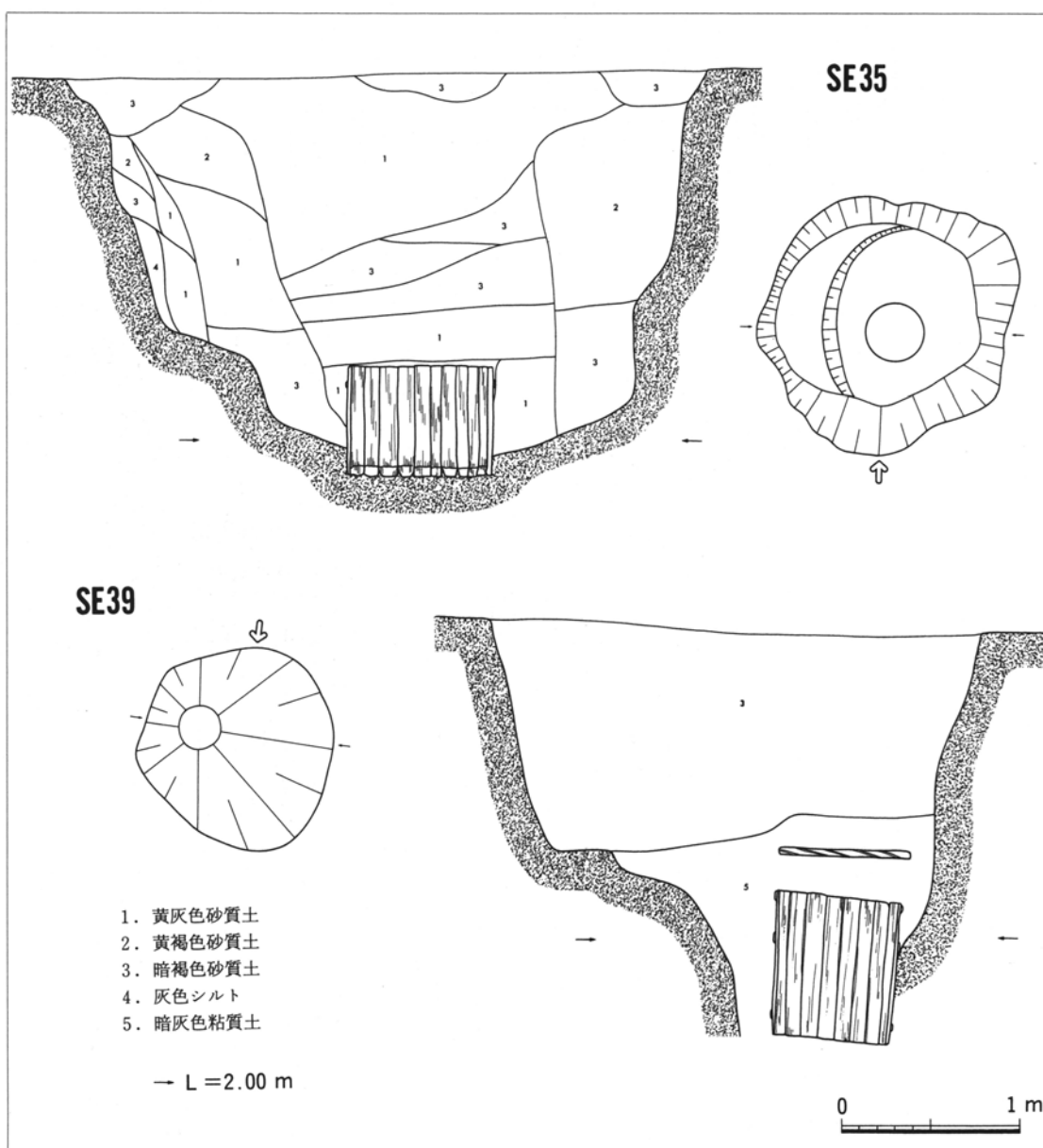
第25図 井戸実測図(10)
