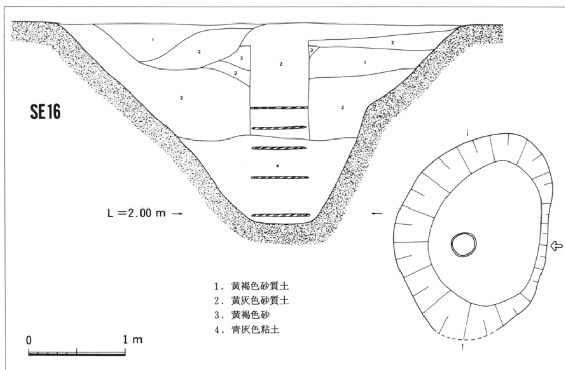
第29図 井戸実測図(14)
