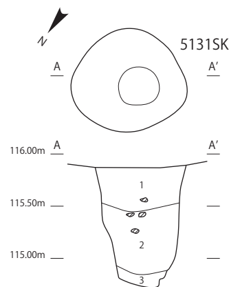
A-A'(5131SK)
