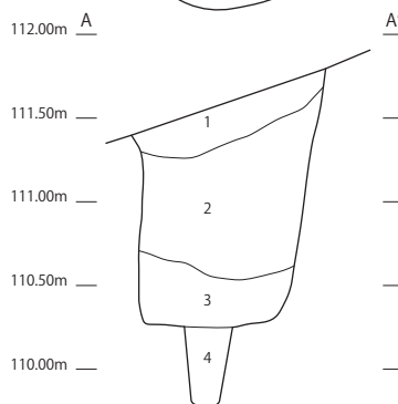
A-A'(3087SK)
