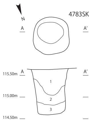
A-A'(4783SK)
