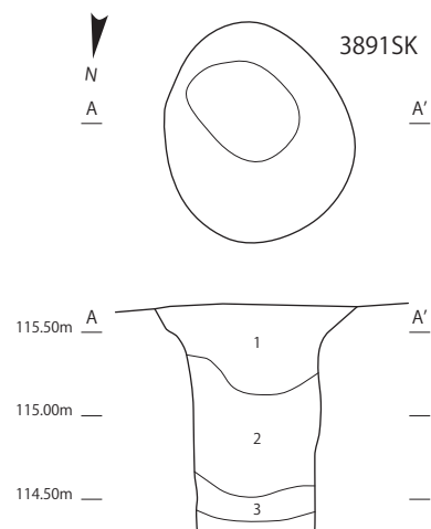
A-A'(3891SK)
