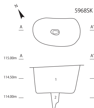
A-A'(5968SK)
