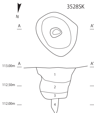
A-A'(3528SK)
