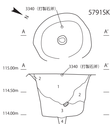
A-A'(5791SK)
