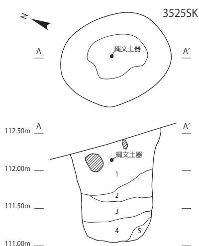
A-A'(3525SK)
