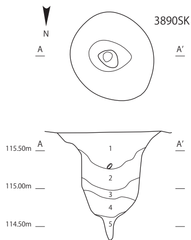
A-A'(3890SK)
