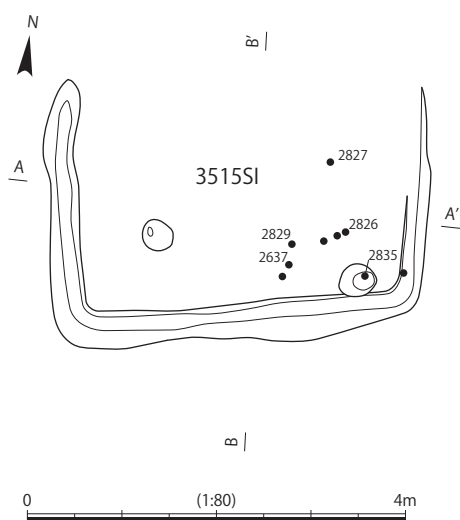
A-A'/B-B'(3515SI)
