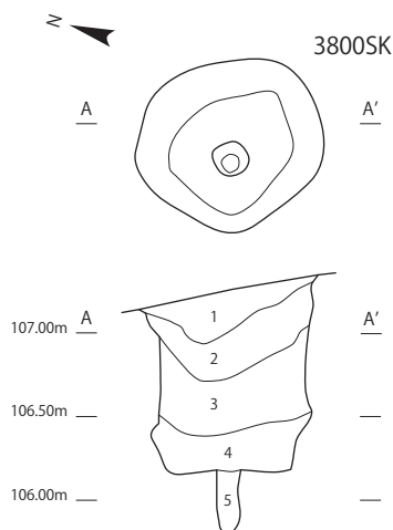
A-A'(3800SK)
