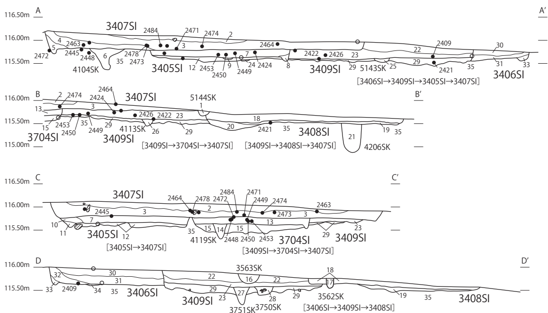
A-A'/B-B'/C-C'/D-D' (3407SI・3405SI・3704SI・3408SI・3409SI・3406SI)
