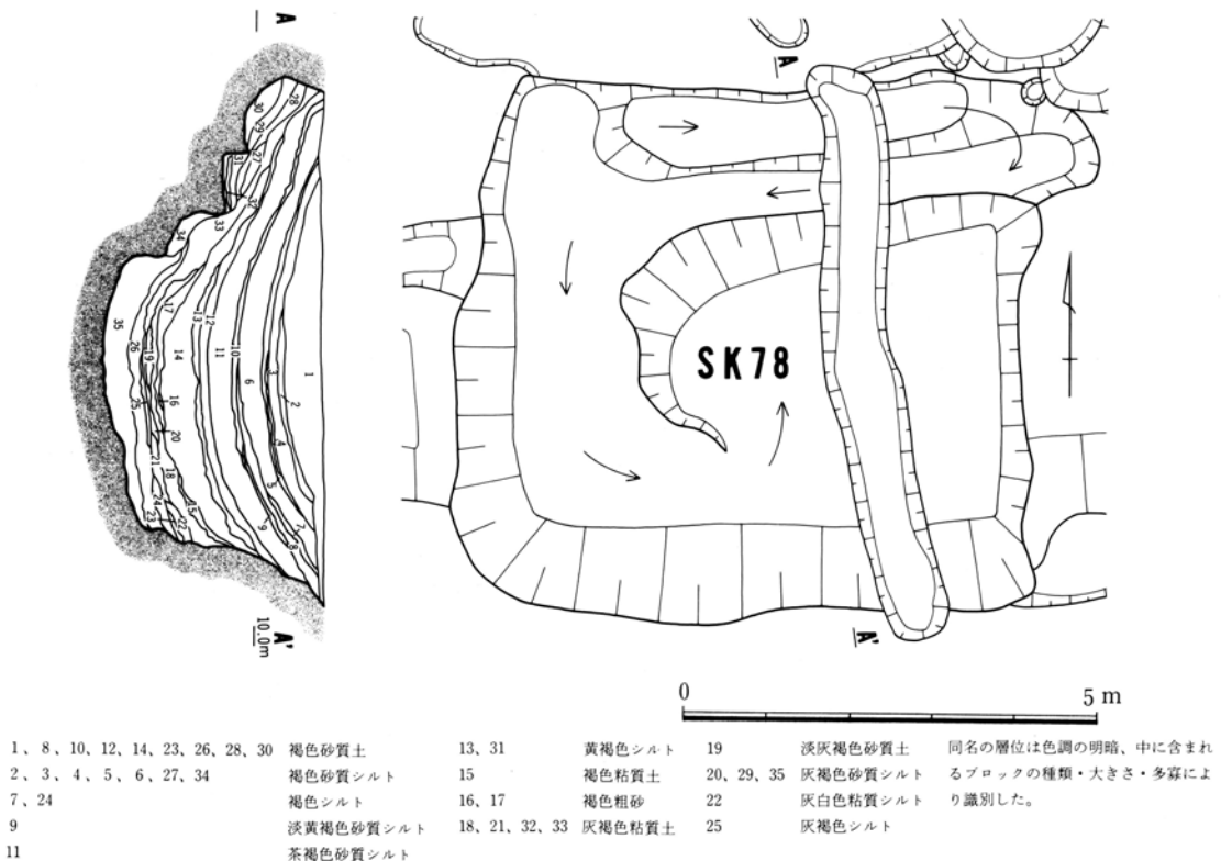
第23図 近世の遺構(9) SK78 平面図・土層セクション (1:100)
