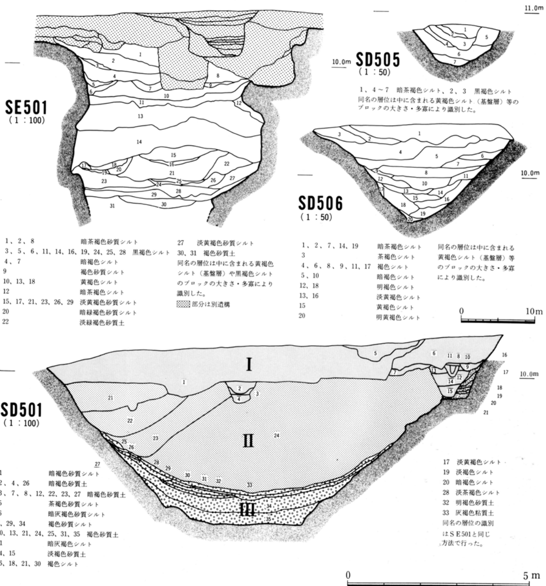
第13図 中世の遺構(3) S D501・505・506、S E501土層セクション (1:50, 1:100)
