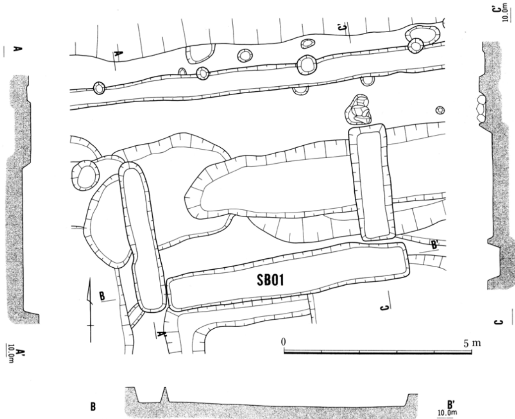
第29図 近世の遺構(15) SB01 平面図・断面図（1：100）
