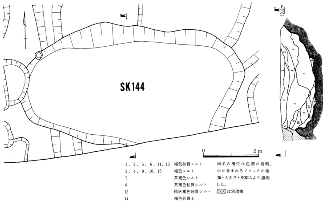
第27図 近世の遺構(13) S K144 平面図・土層セクション (1 : 80)
