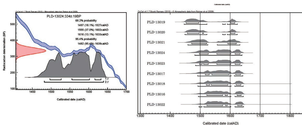
第 98 図 漆器椀 (試料 No.126(4)) の塗膜の暦年校正図とマルチプロット図
