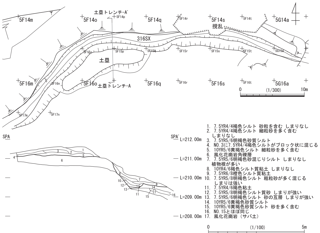
第 31 図 08 A 区 土塁トレンチ
