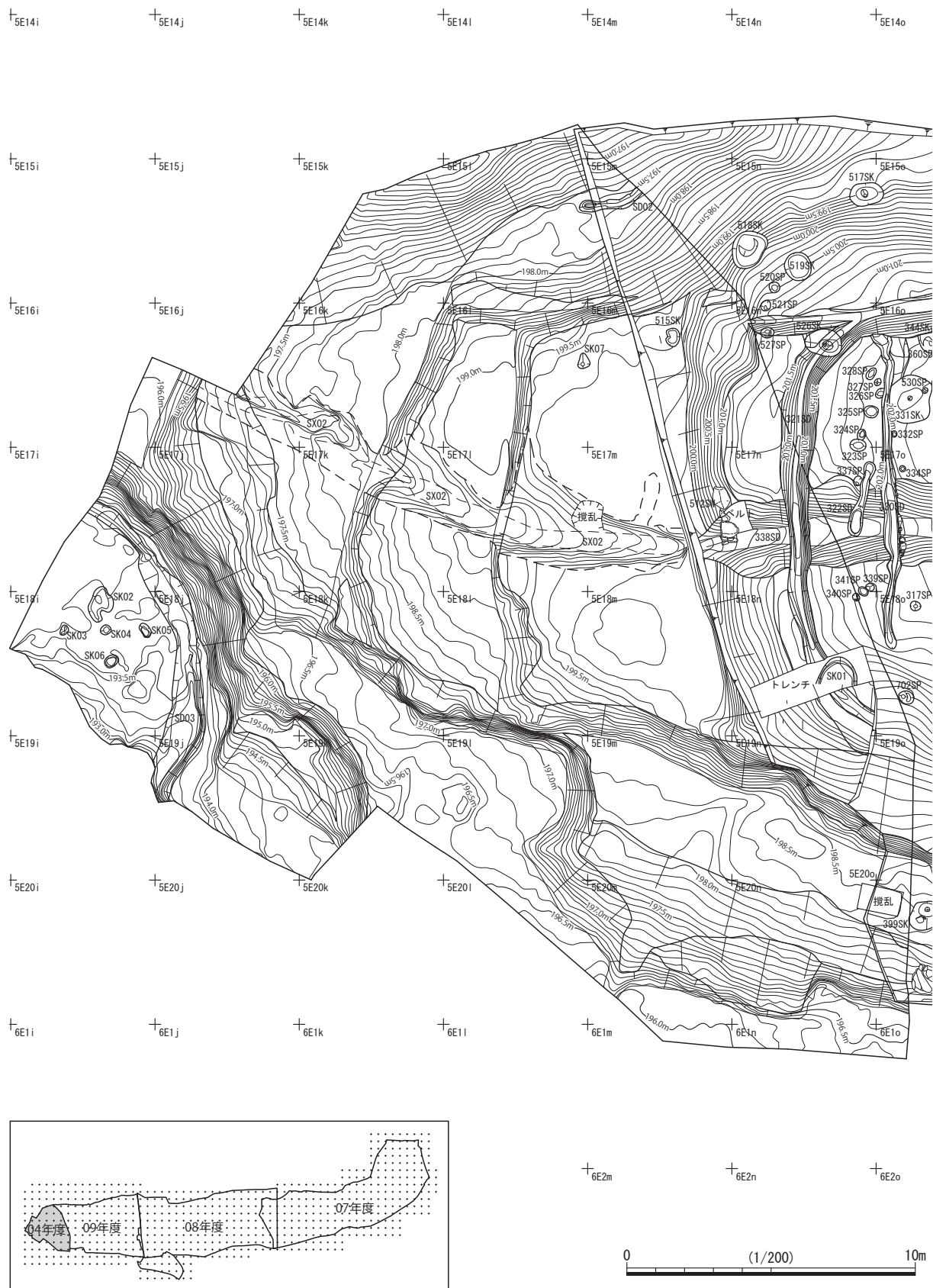
第 7 図 04 調査区全体図 (1:200)
