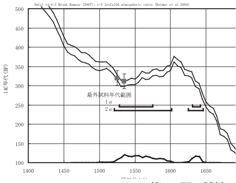
第 93 図 試料 No.5：ウィグルマッチング結果
