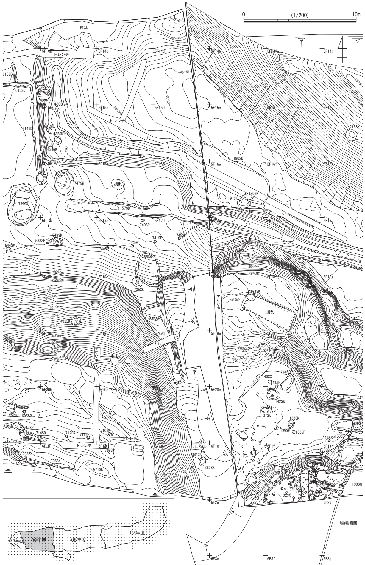
第 9 図 09 調査区全体図 (1:200)
