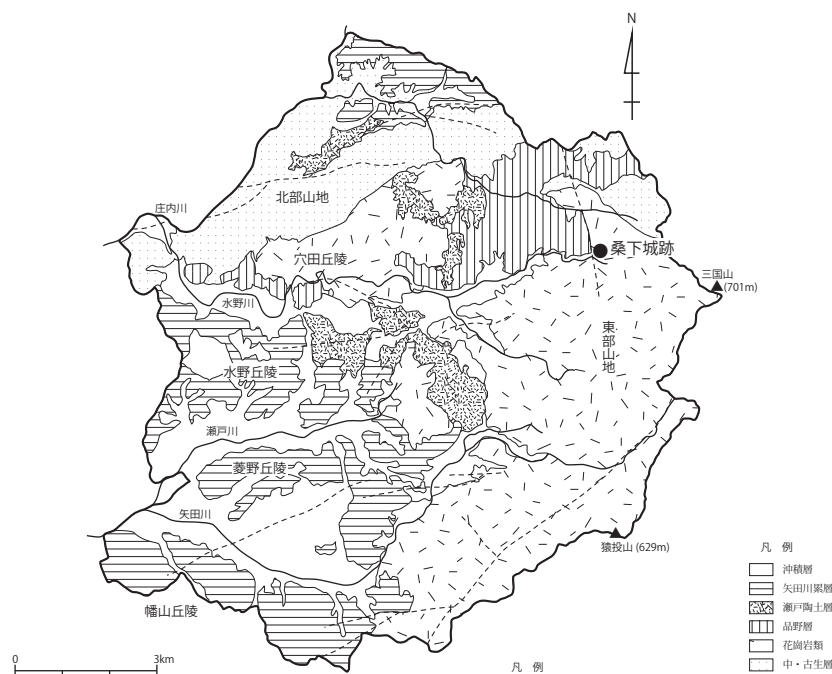
第2図 瀬戸市の地質概要図 『瀬戸市史』自然編をもとに作成
