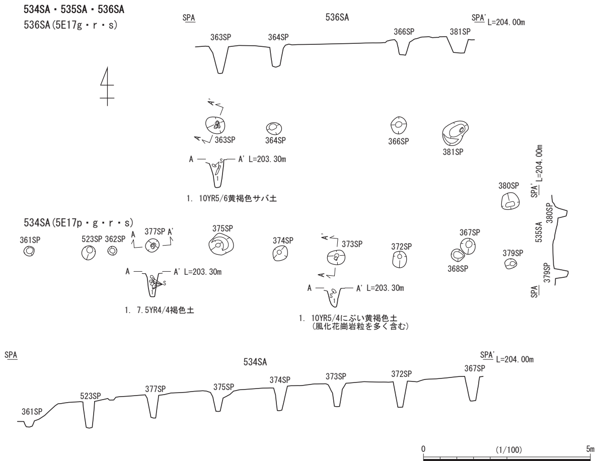
第20図 09区 534SA・535SA・536SA(1:100)
