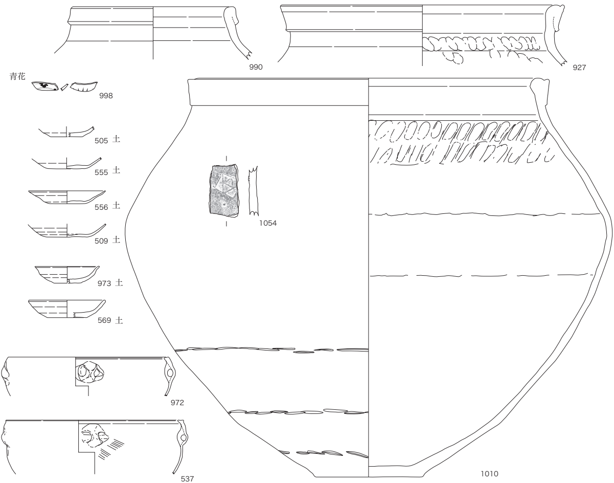
第 112 図 中世に搬入された遺物 (1) (S=1/6)
