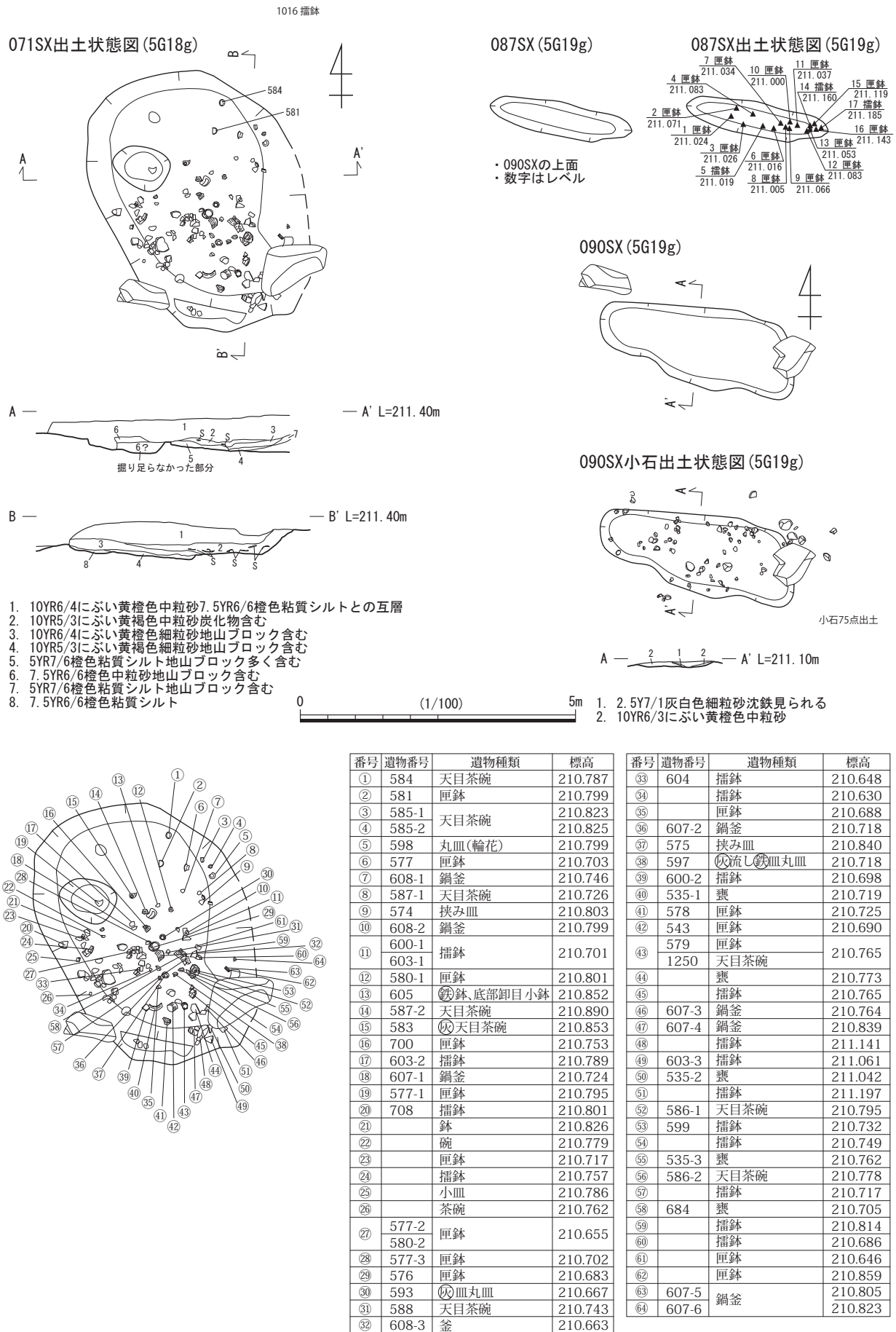
第 52 図 07 A 区 071SX・087SX・090SX(1:100)
