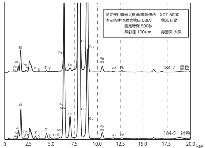
第 106 図 184 小刀 表面のスペクトル図
