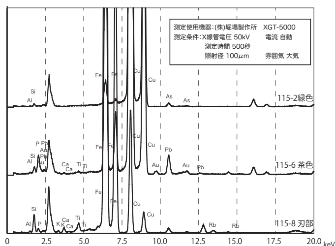
第 104 図 115 小刀 表面のスペクトル図
