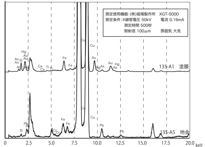
第 105 図 135 簪 表面のスペクトル図
