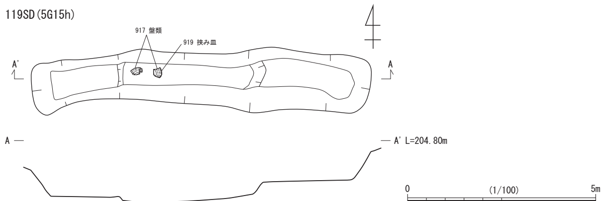
第 55 図 07 A 区 119SD(1:100)
