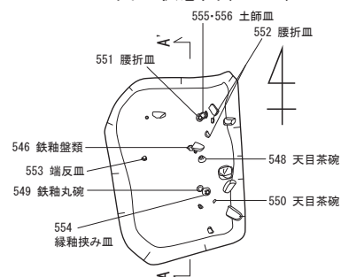
006SX出土状態図 (5G19f)
