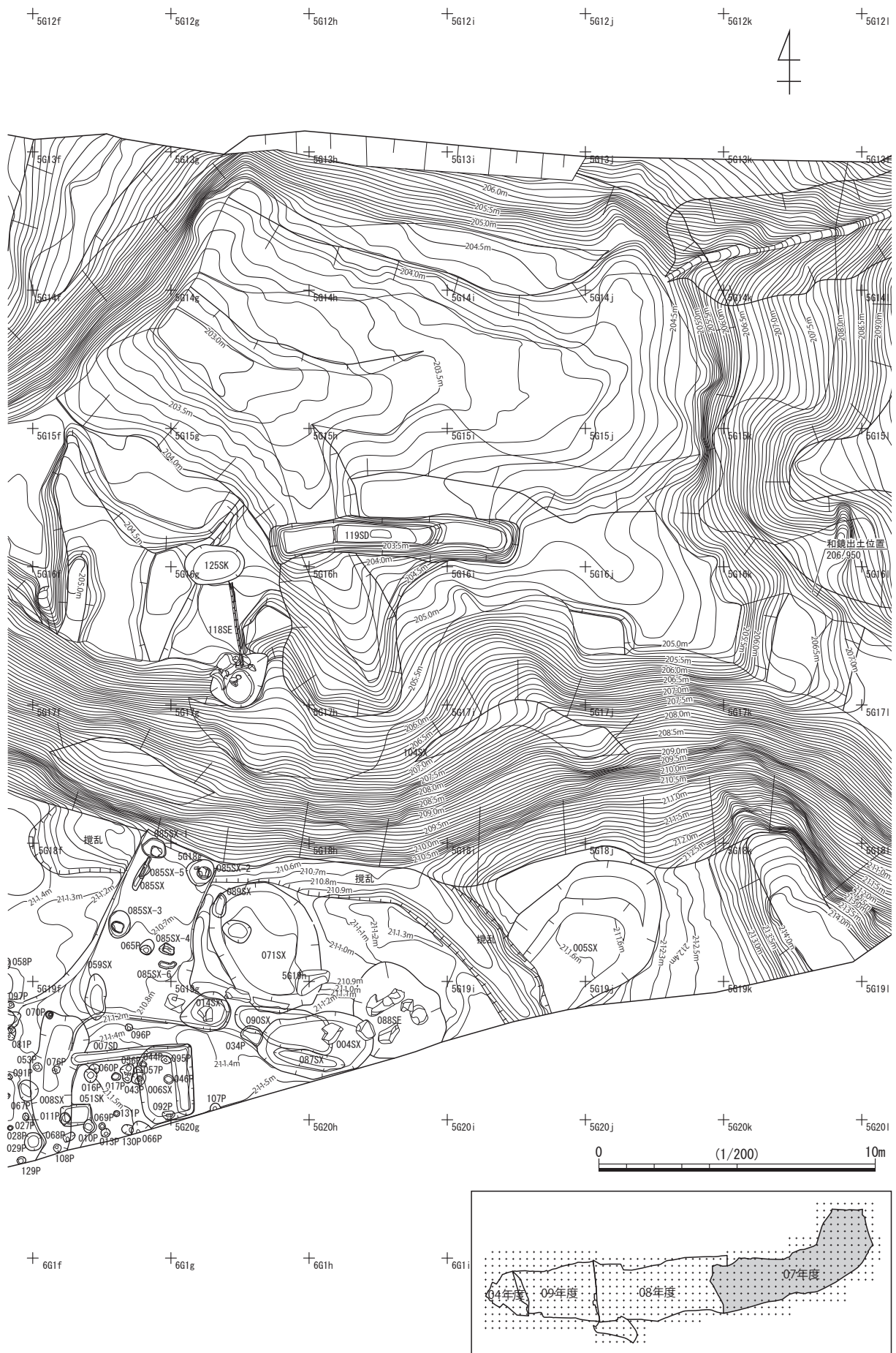
第 13 図 07 調査区全体図 (1:200)
