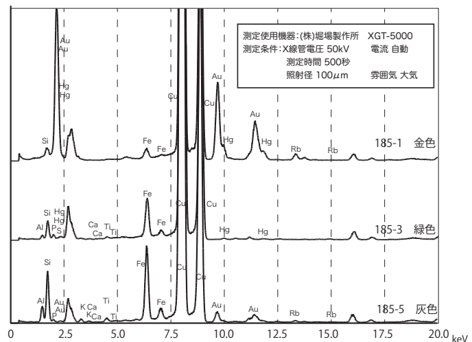
第 107 図 185 飾り金具 表面のスペクトル図
