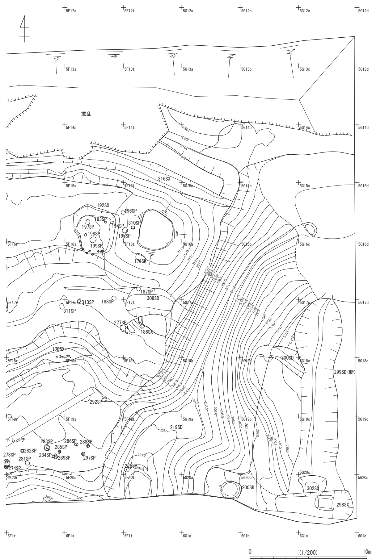
第 43 図 07 A 区 299SD (新) (1:200)
