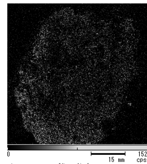
▲ 004SX 鉛の分布
