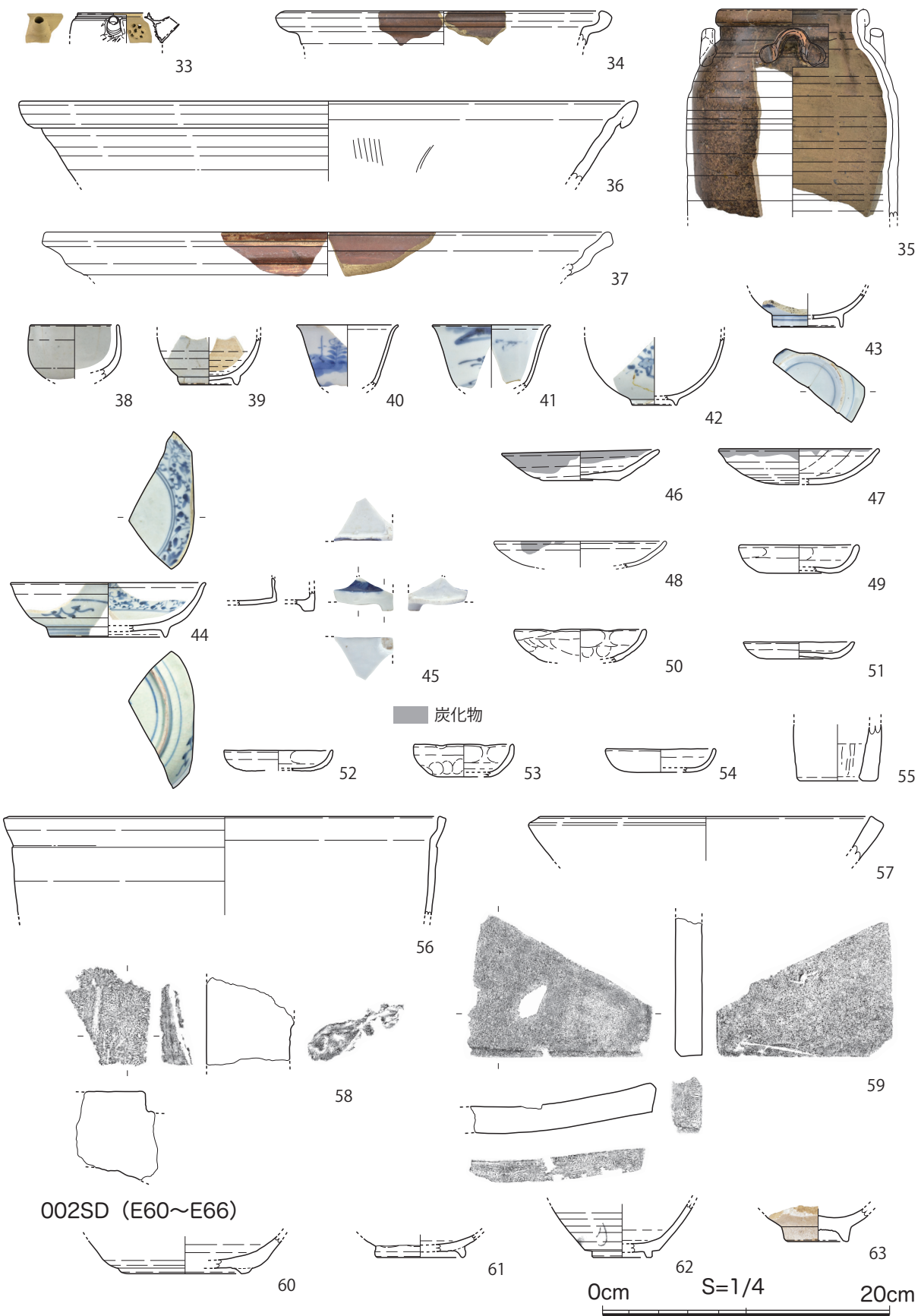
図 10 出土土器・陶磁器 2 (1 : 4)
