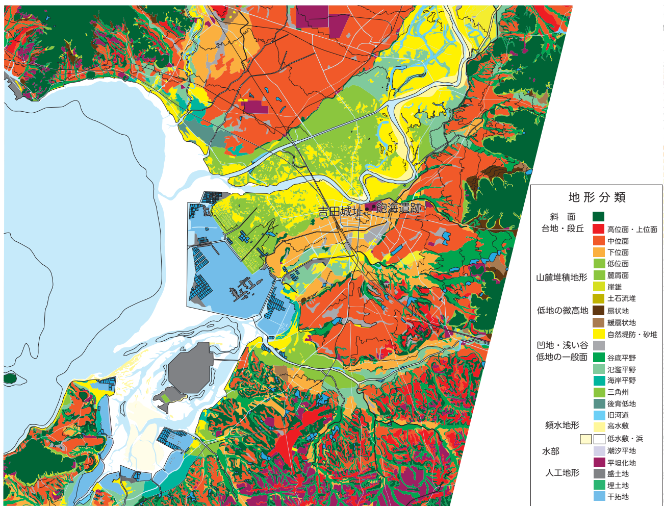
図 15 吉田城址・飽海遺跡の立地 (1:100,000)
