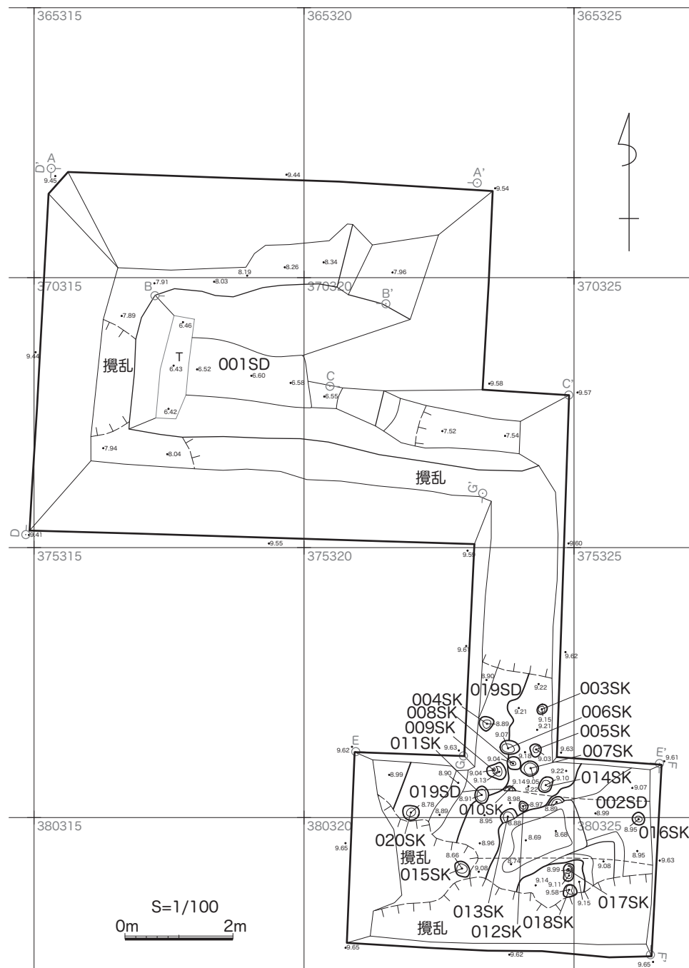
図4 遺構平面図 (1:100)
