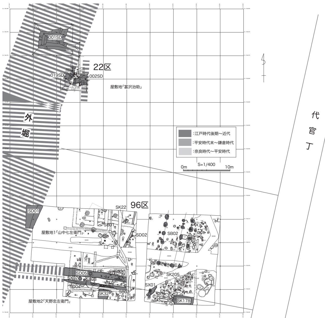
図13 22区・96区遺構変遷図(1:400)
