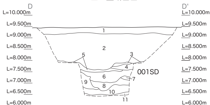
22A区西壁断面図
