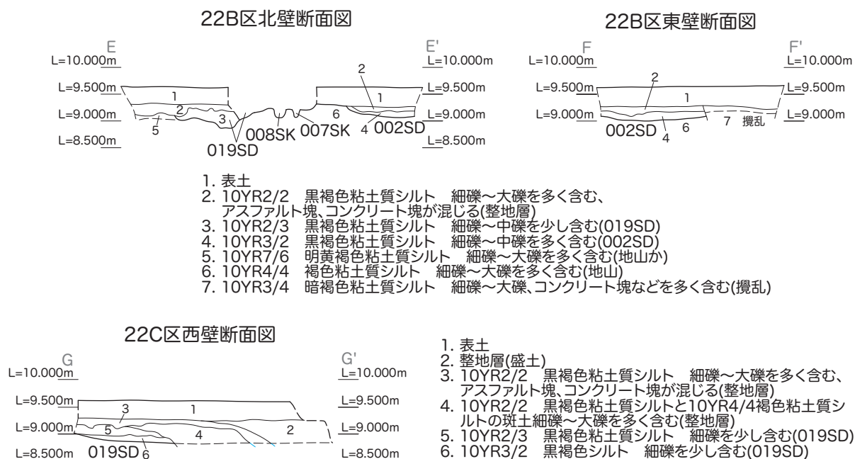
図6 基本層序2 (1:100)
