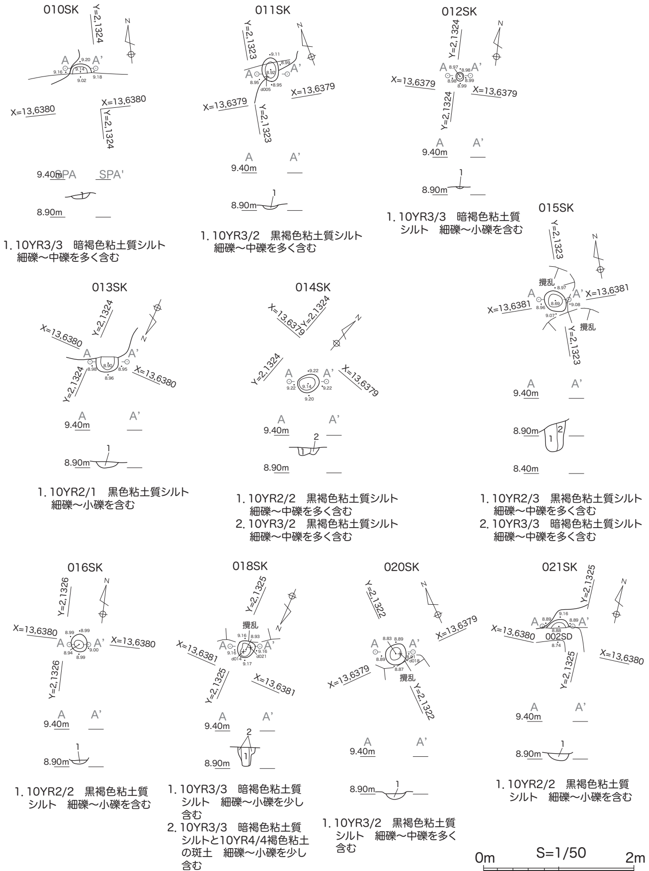
図8 個別遺構図2 (1:50)
