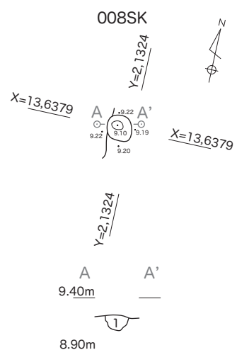
図7 個別遺構図1 (1:50)
