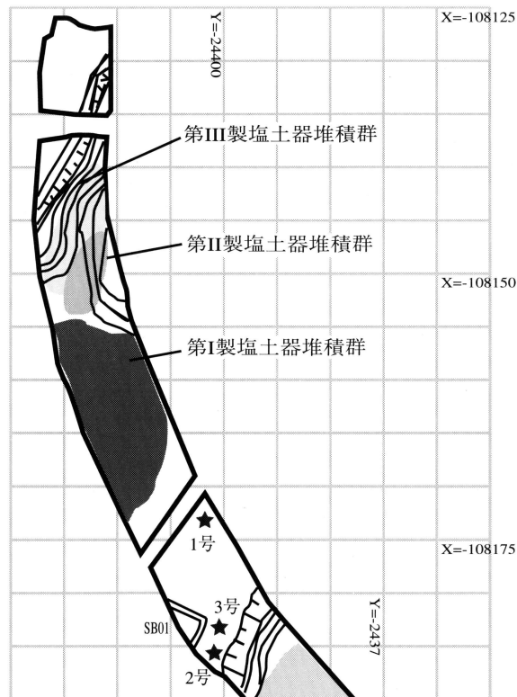
第1図 松崎遺跡遺構配置図
