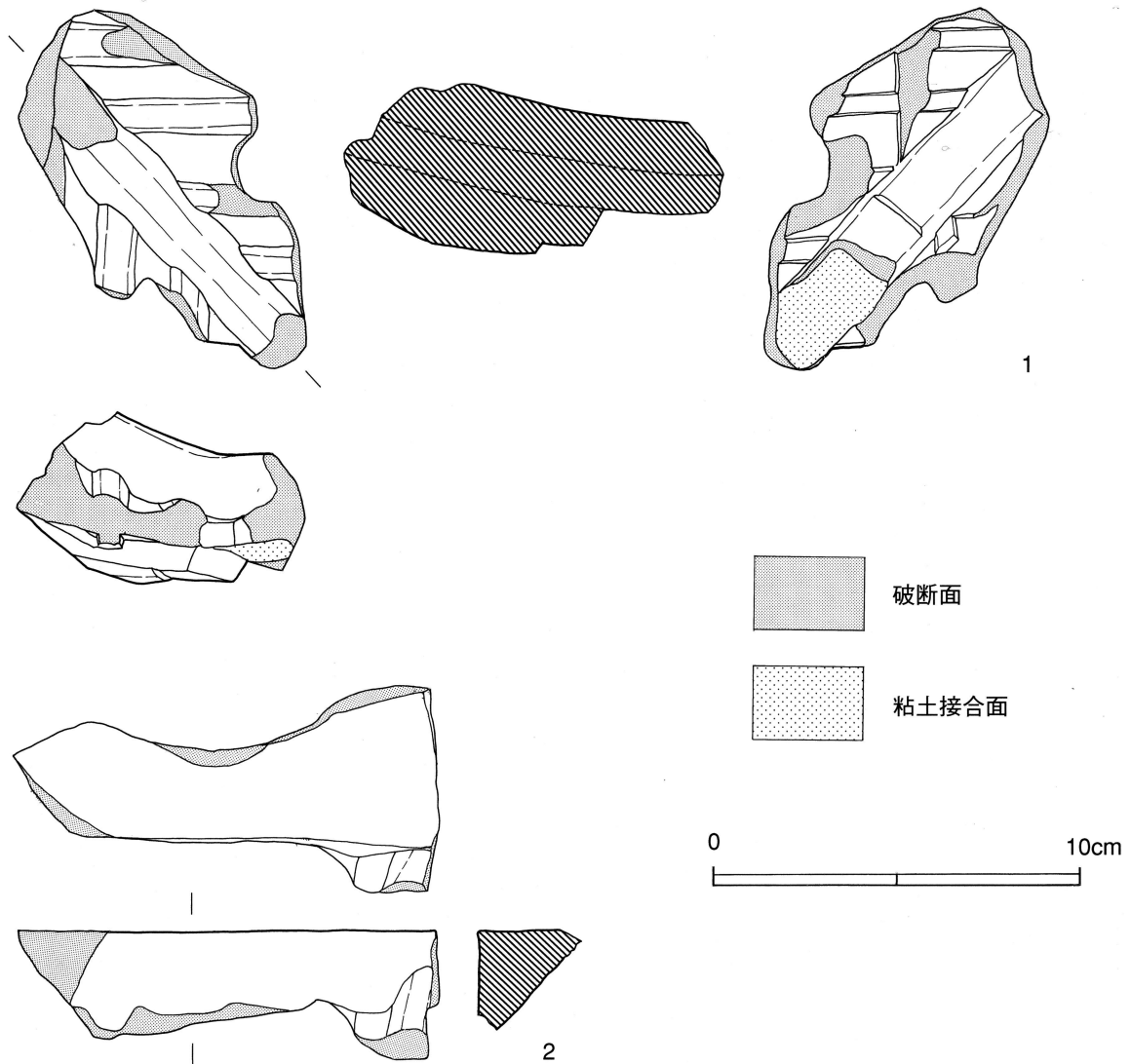
第4図 瓦塔屋蓋部実測図② (1:2)
