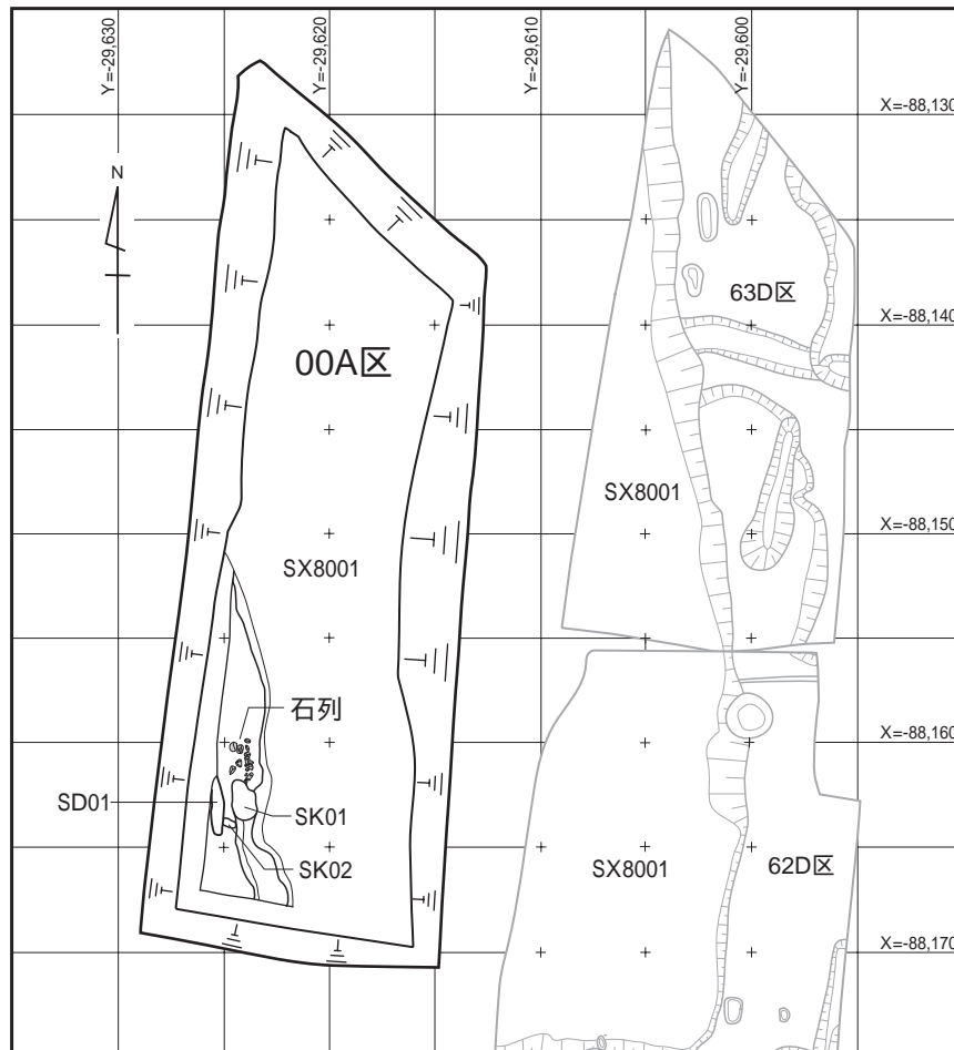
00 A 区遺構図 ( 1 : 400 )
