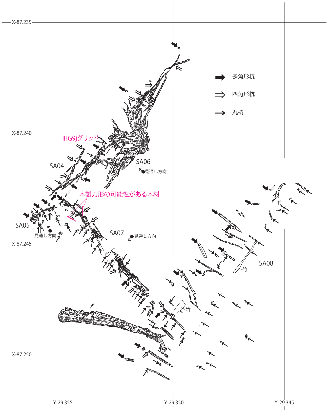
図2 木製刀形出土状態図 (1/80 報告書第15図を一部改変)
