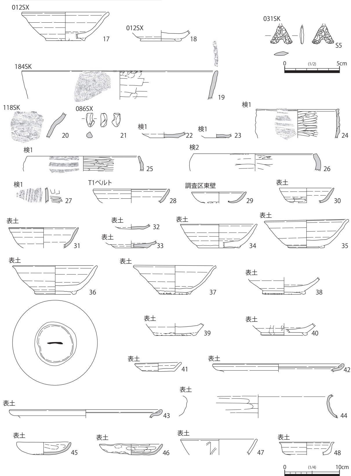
図 24 08Ba 区出土遺物実測図 (1)
