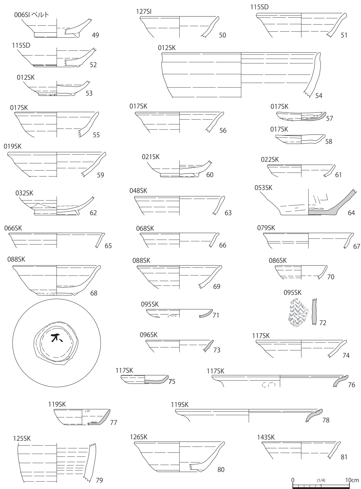
図 26 08Bb 区出土遺物実測図 (1)
