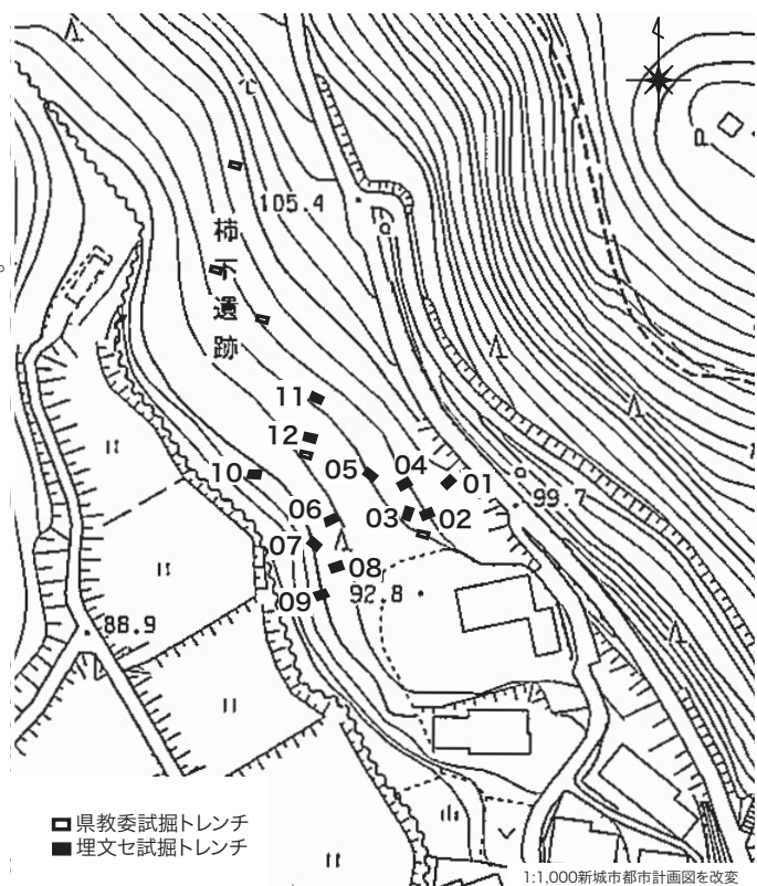
図5 試掘トレンチ配置図
