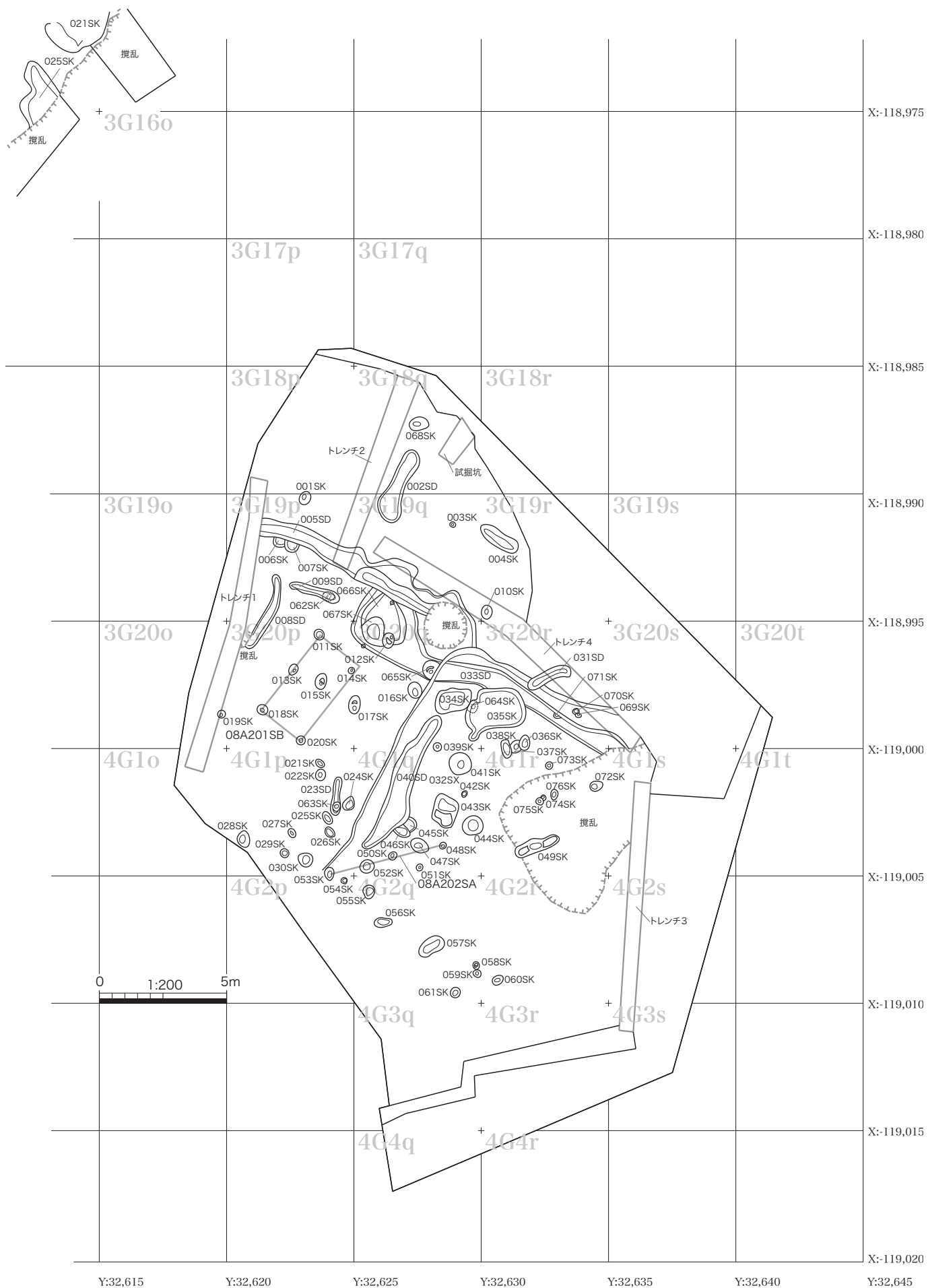
図 42 柿下遺跡 A 区基本遺構平面図
