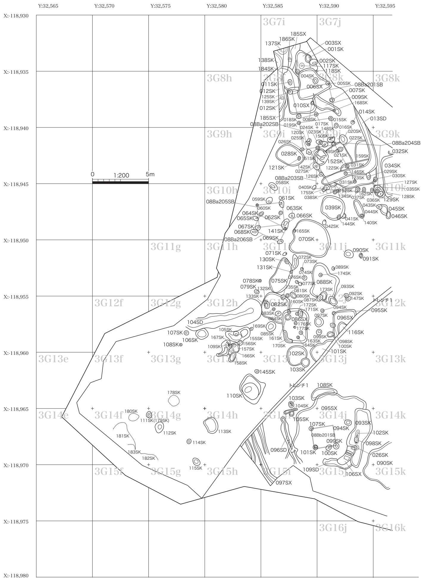
図 40 柿下遺跡 B 区基本遺構平面図 (1)
