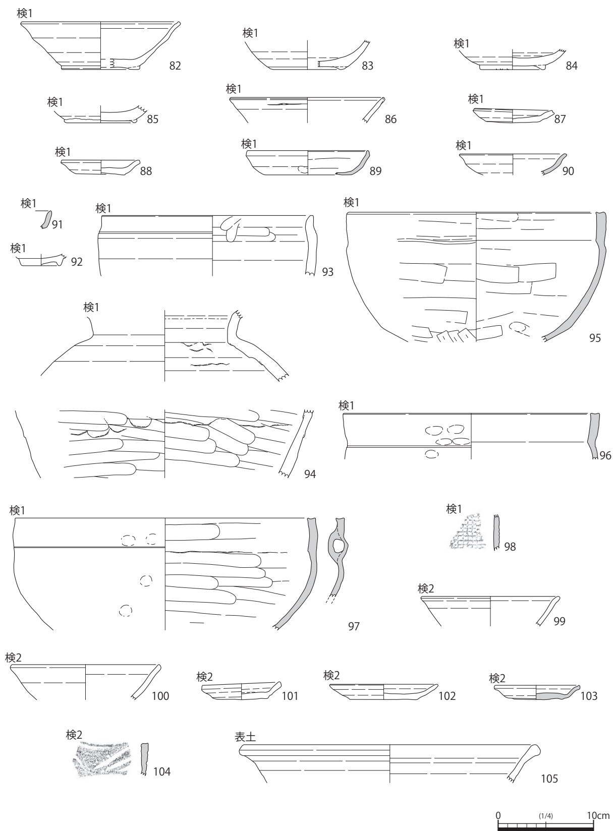
図 27 08Bb 区出土遺物実測図 (2)
