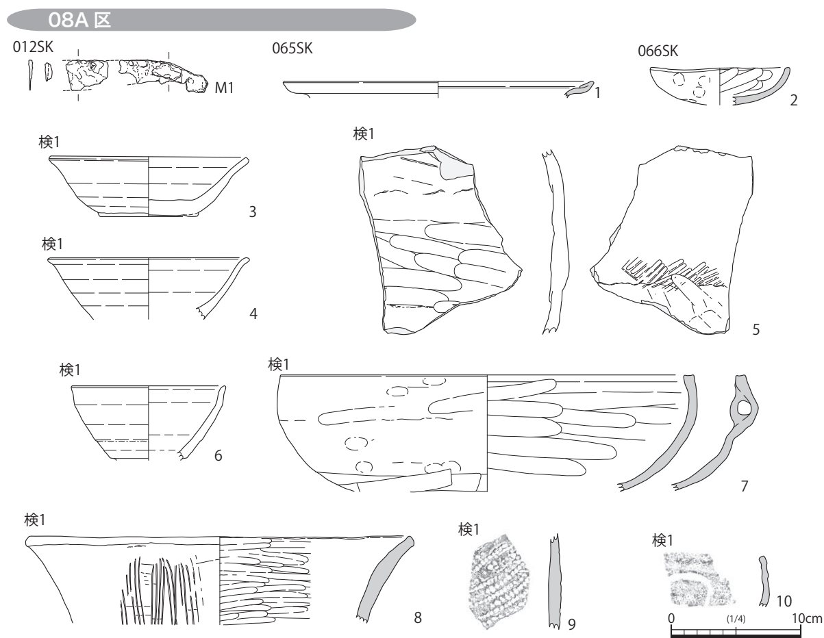
図22 08A区出土遺物実測図(1)
