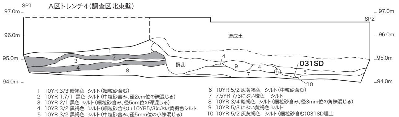
図 13 基本土層断面図 (08A 区)
