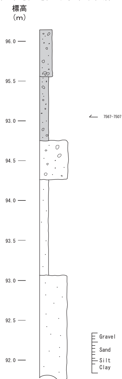
図 31 地点 2 柱状図
