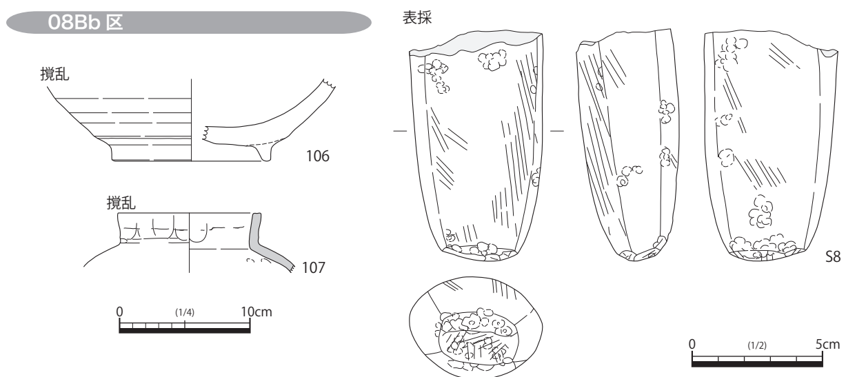
図 28 08Bb 区出土遺物実測図（3）
