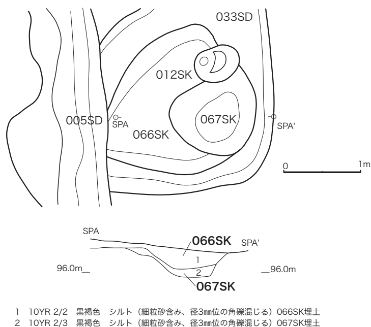
図 14 08A 区 066SK・067SK 遺構図
