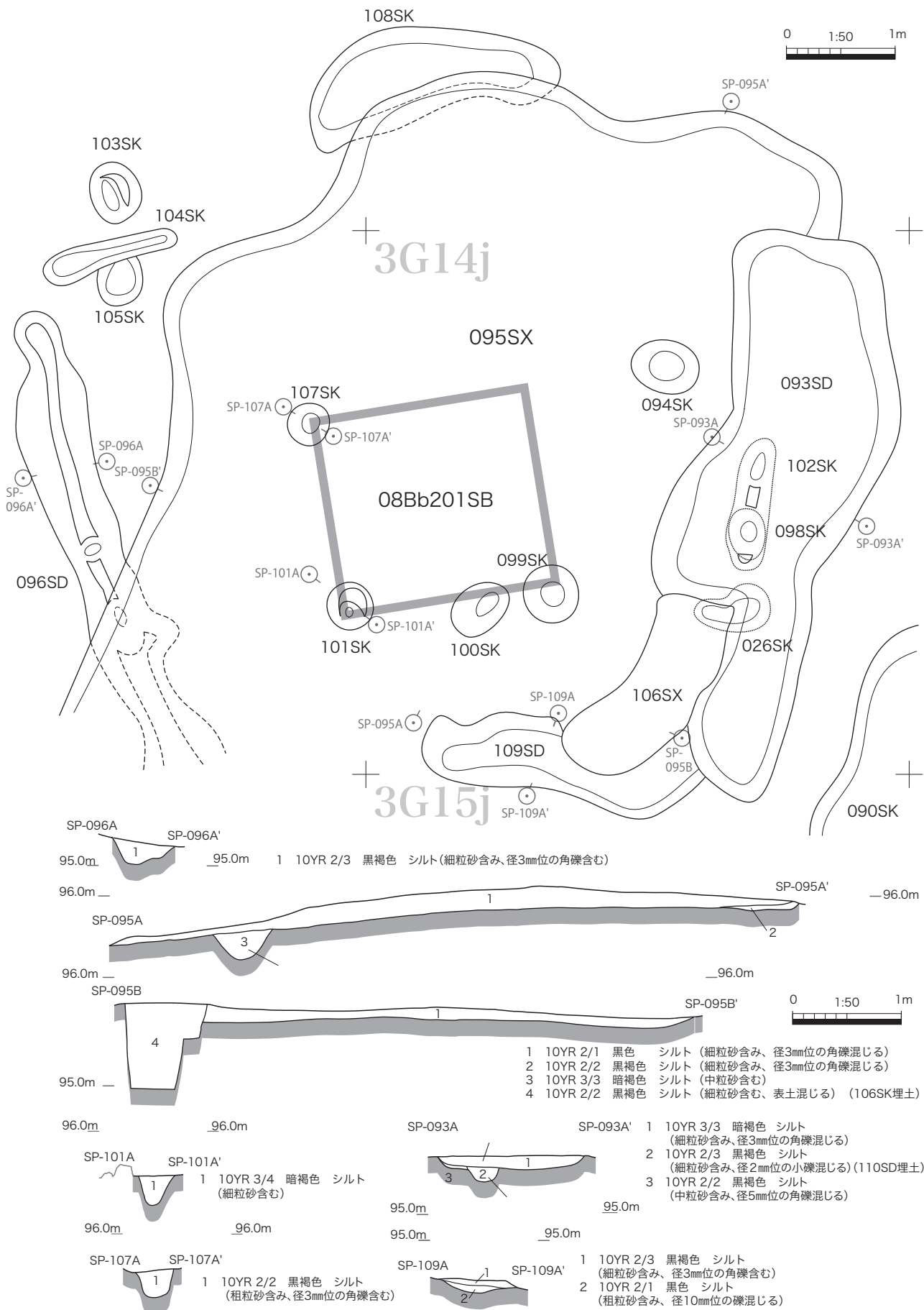
図 20 08Bb 区 095SX 遺構図
