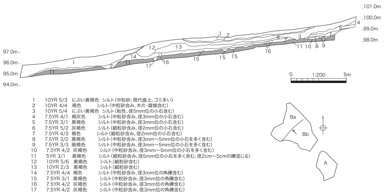
図12 基本土層断面図（08Ba区）
