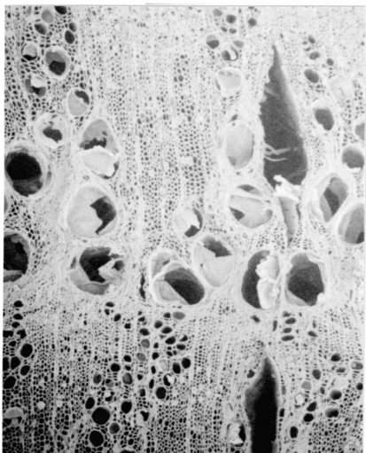
2a クリ (横断面) No. 15 1.0mm
