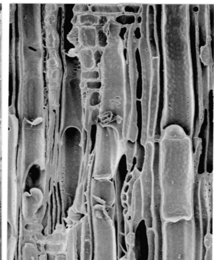
2c クリ (放射断面) No. 15 0.1mm
