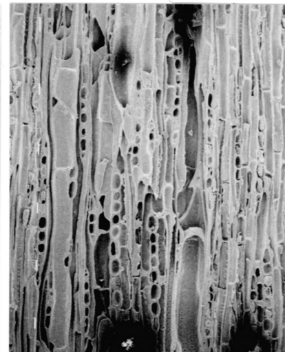
2b クリ (接線断面) No. 15 0.1mm
