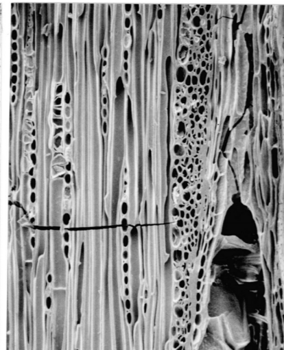
3b ツブラジイ (接線断面) No. 10 0.1mm
