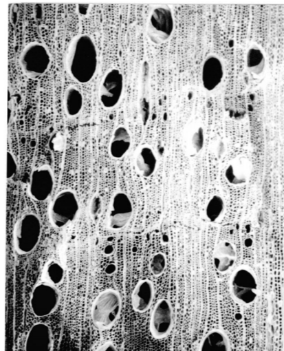
4a シイノキ属 (横断面) No. 3 1.0mm
