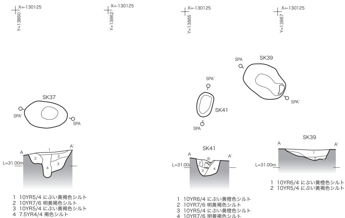
第16図 SK39・SK41平・断面図 (1/50)
