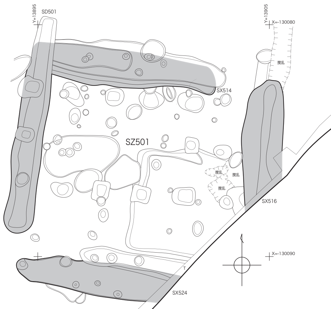
第34図 S Z501平面図 (1/100)
