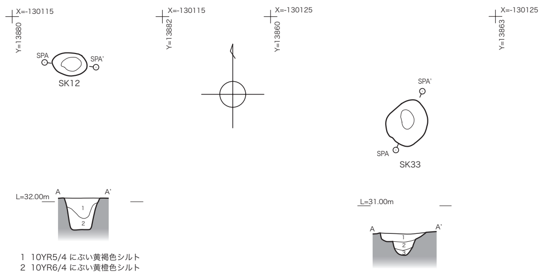
第13図 SK12平・断面図 (1/50)
