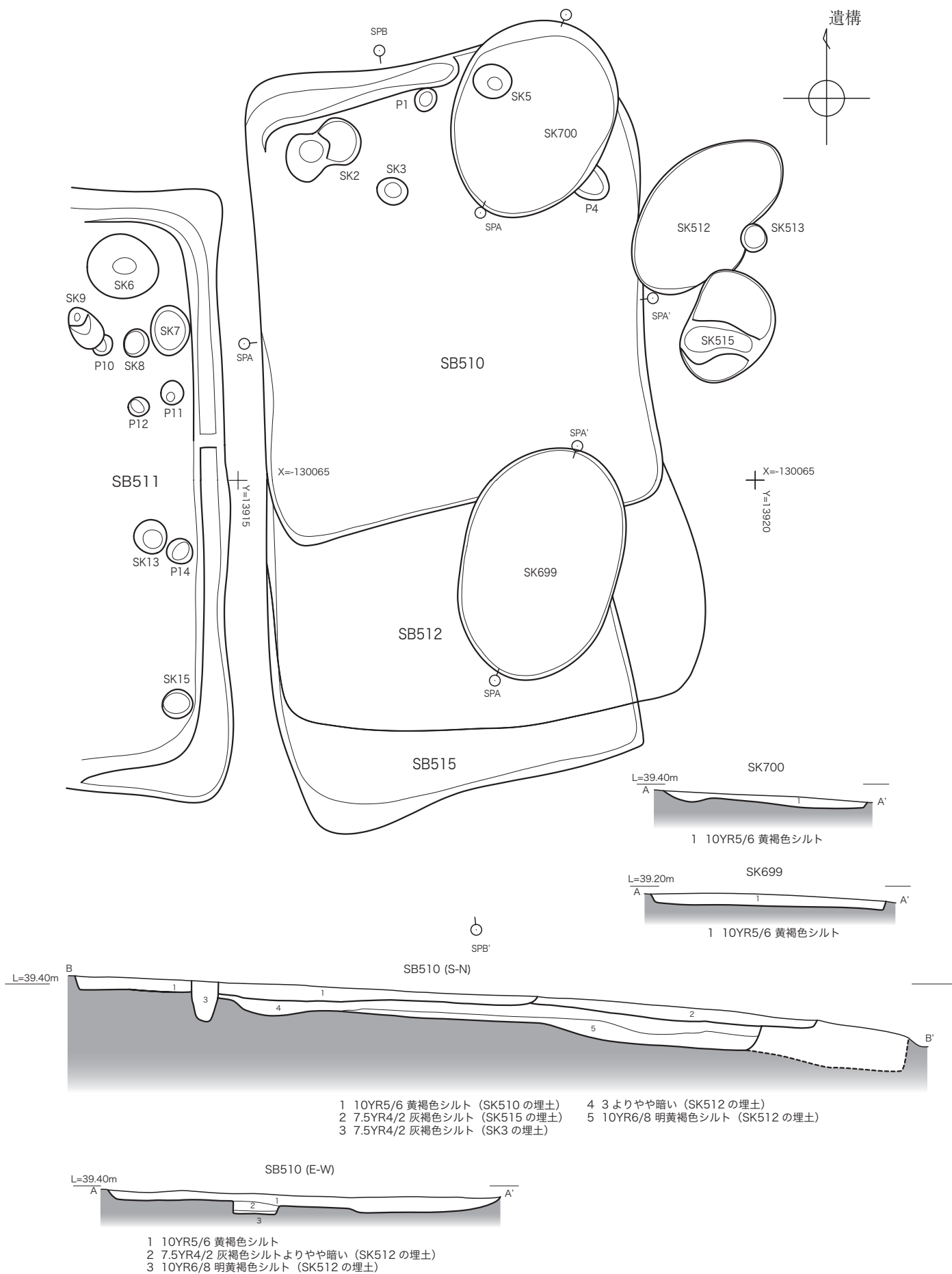
第24図 SB510・515平・断面図 (1/50)
