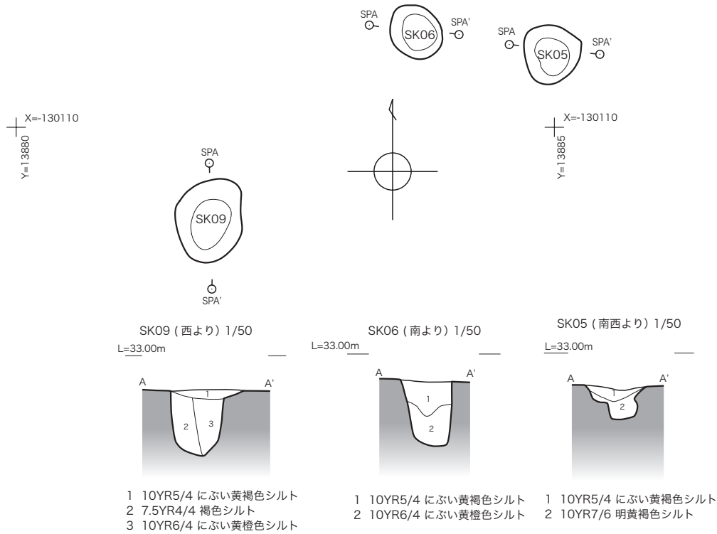
第10図 SK05・06・09平・断面図 (1/50)
