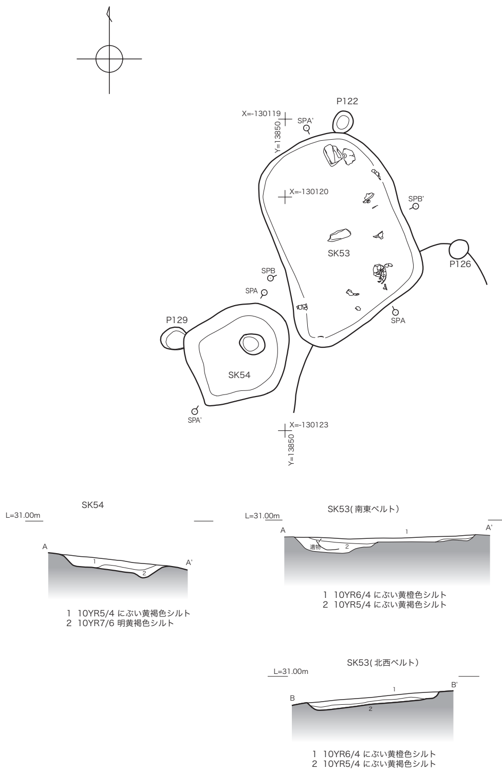
第17図 S K53・54平・断面図 (1/50)
