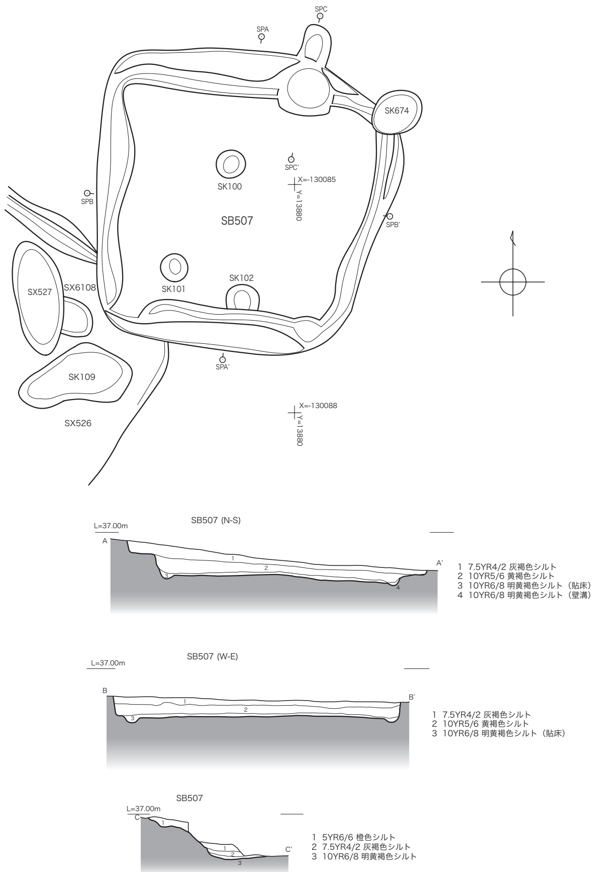
第21図 S B 507平・断面図 (1/50)
