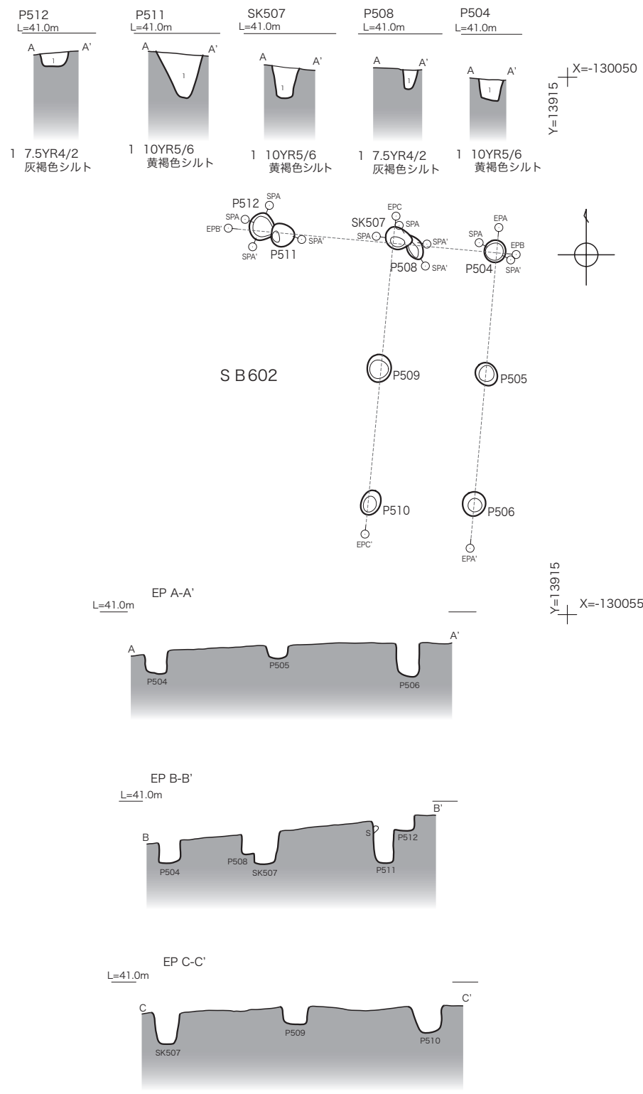
第27図 S B 602平・立面図 (1/50)
