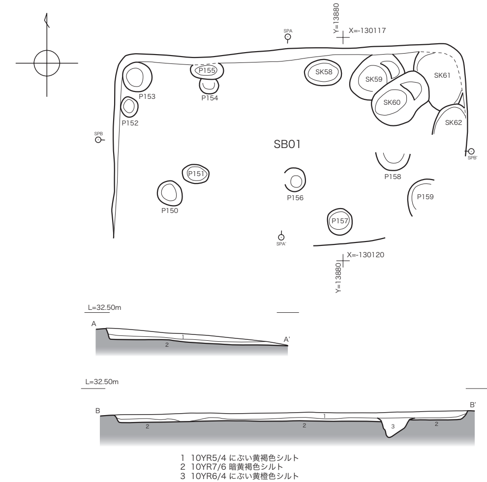
第9図 SB01平・断面図 (1/50)
