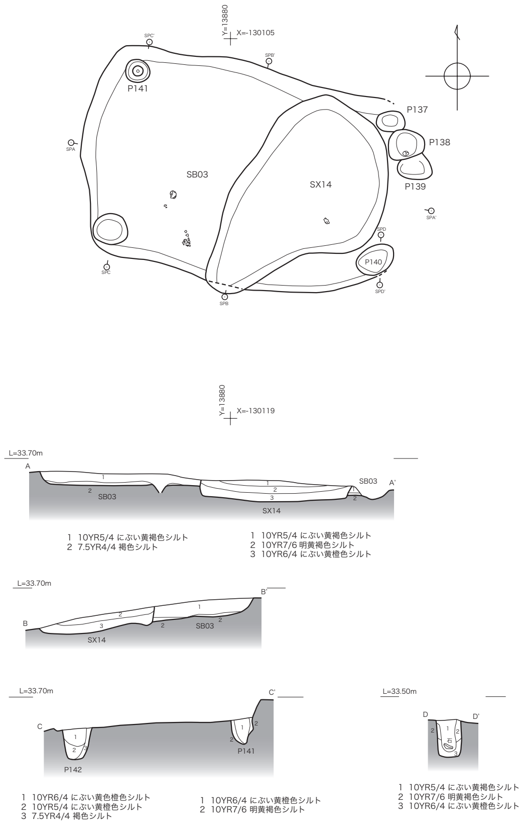
第12図 S B03・S X14平・断面図 (1/50)
