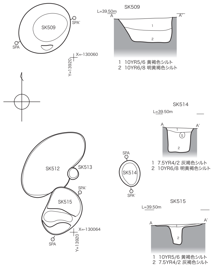
第28図 S K 509・514・515平・断面図 (1/50)
