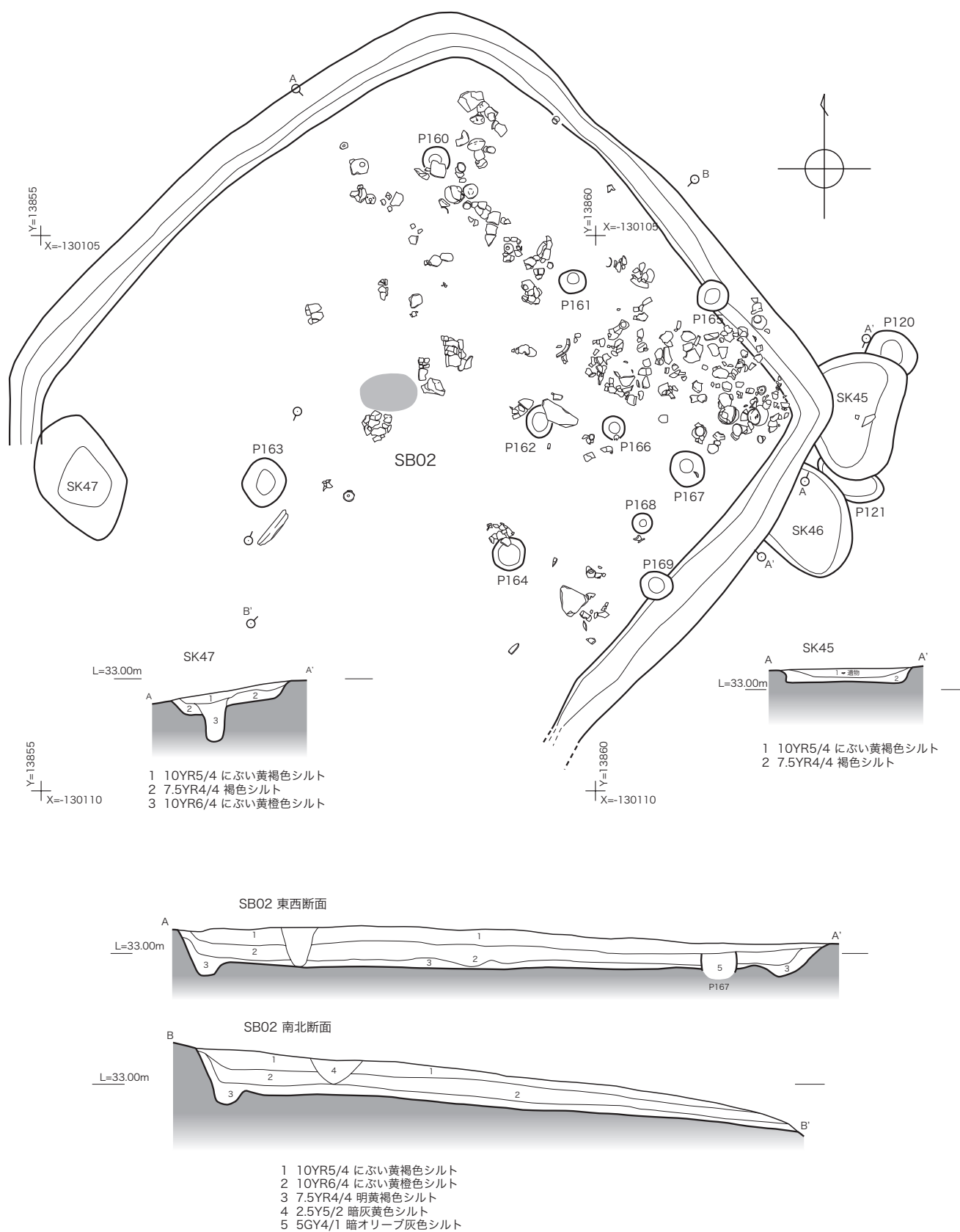
第11図 SB02・SK45・47平・断面図 (1/50)
