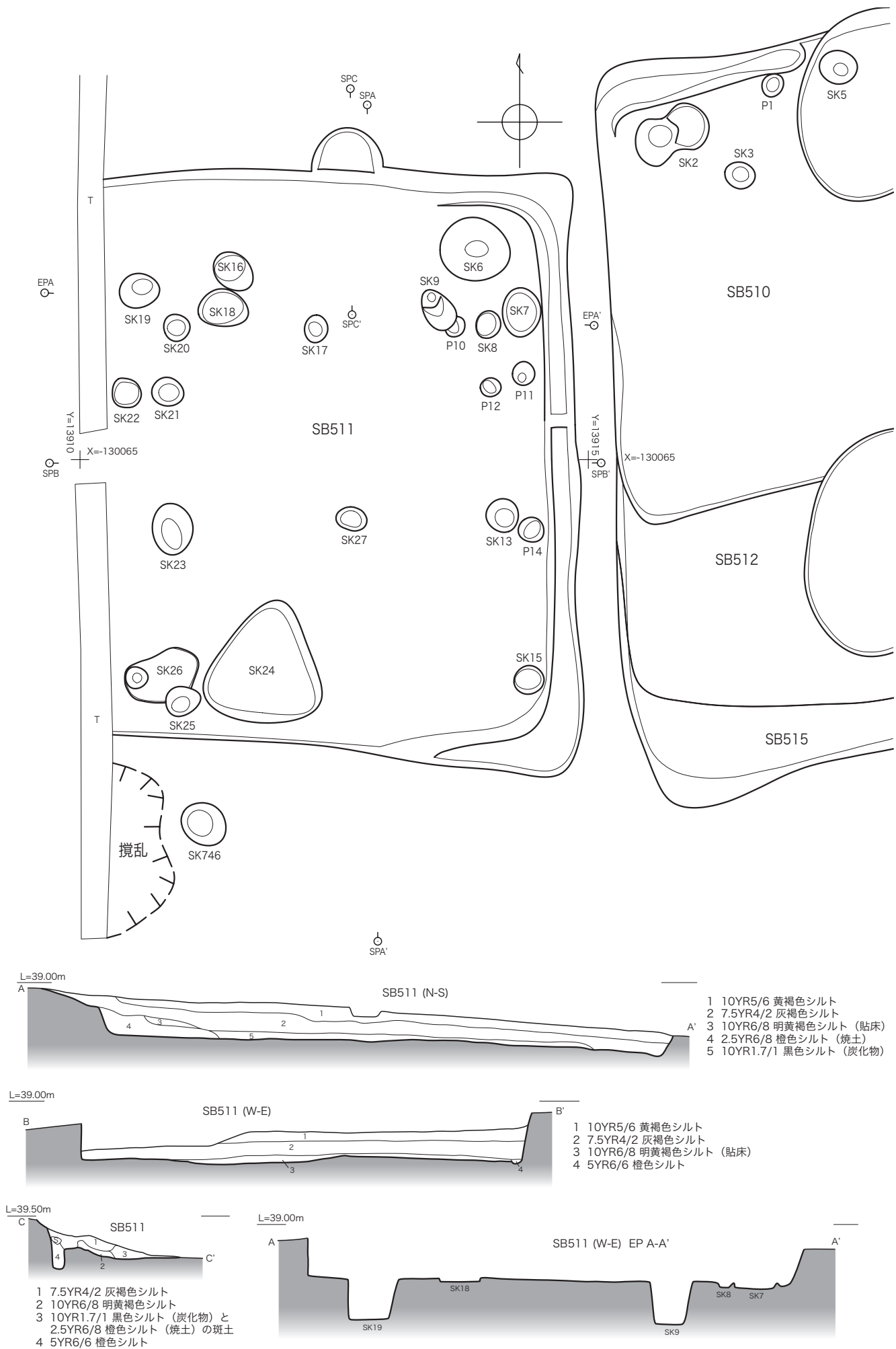
第25図 SB511平・断面図 (1/50)
