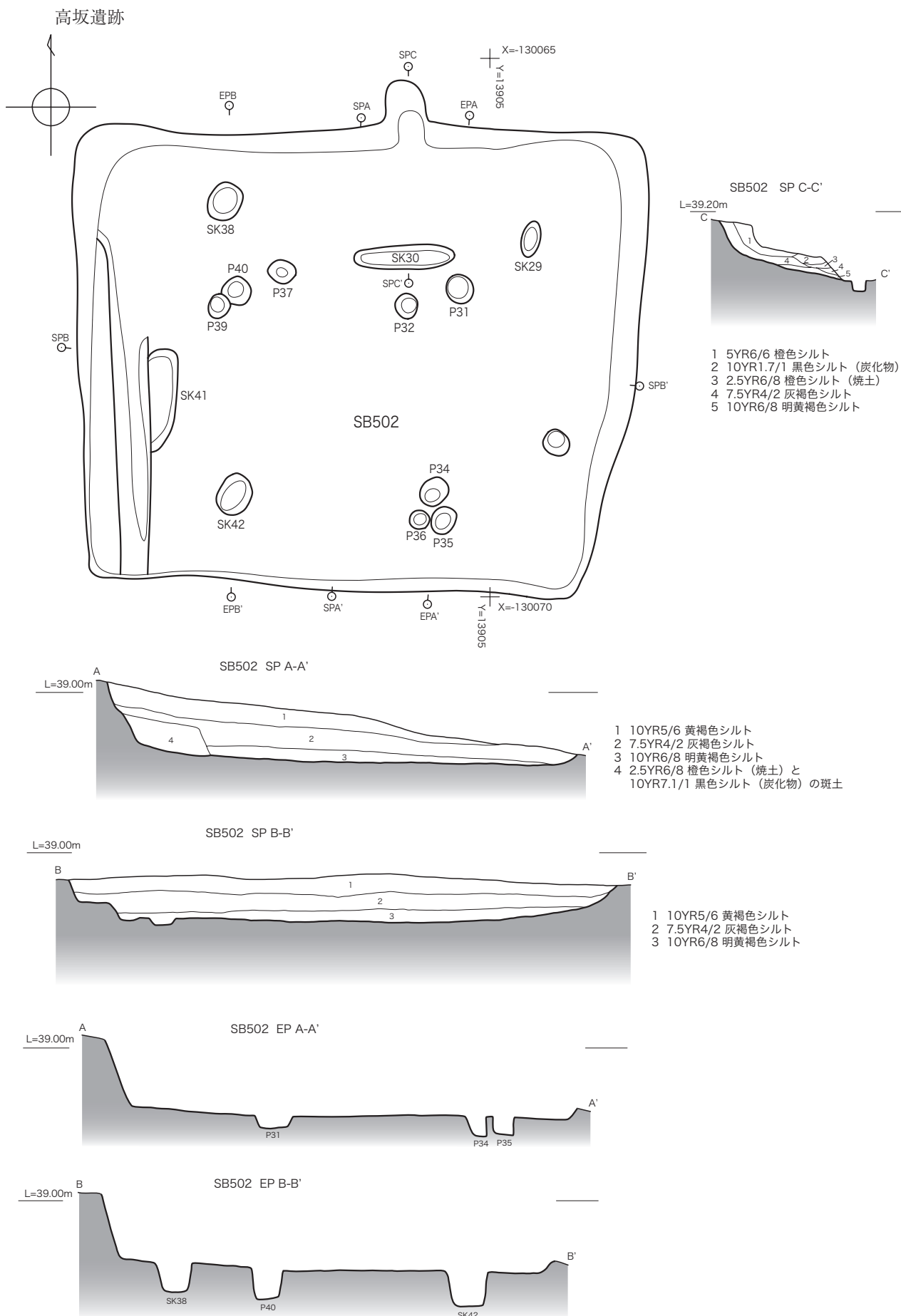
第19図 SB502平・断面図 (1/50)
