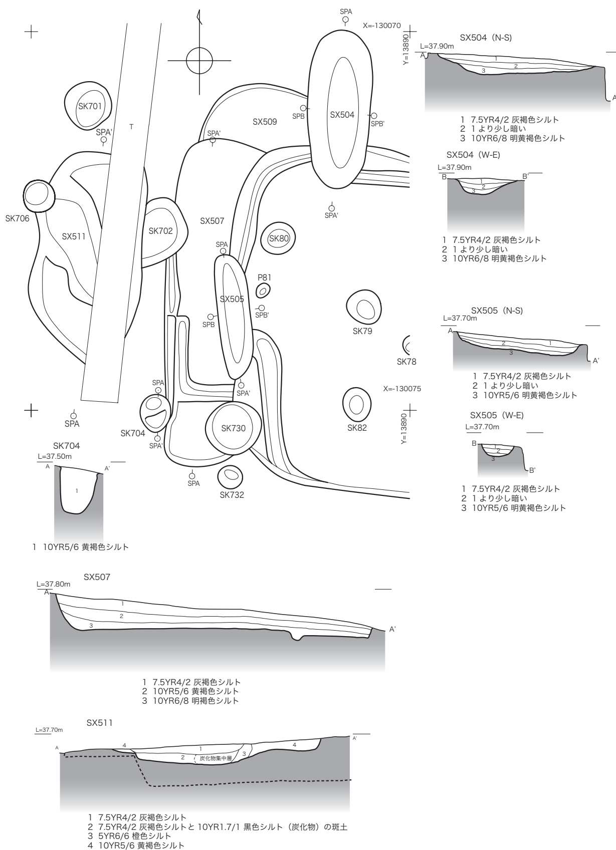
第31図 S X504・507・511・S K704平・断面図 (1/50)
