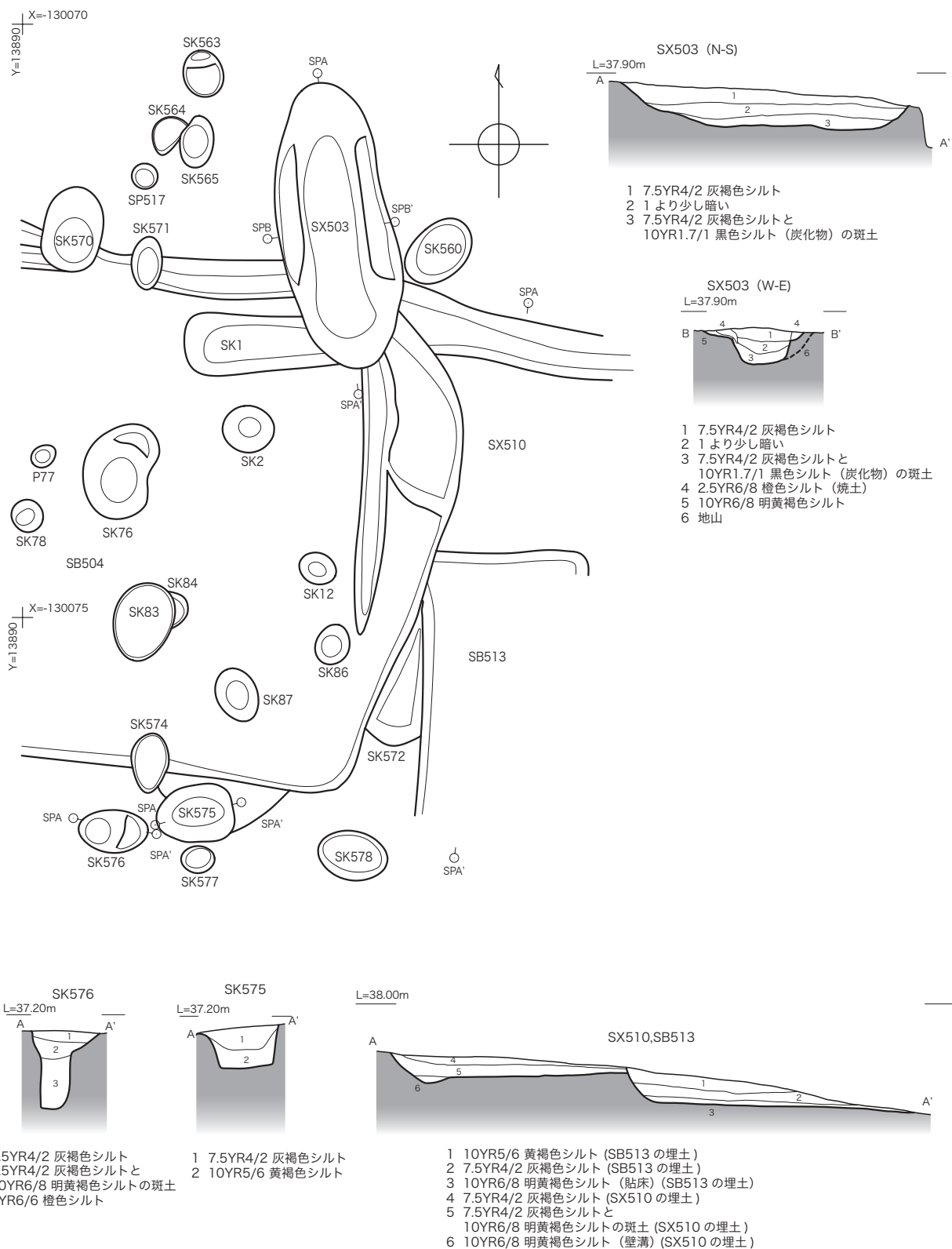
第30図 S X 503・510・S K 575・576平・断面図 (1/50)
